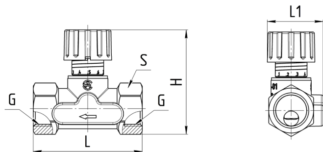
Рисунок 3 – Габаритные размеры клапана.
