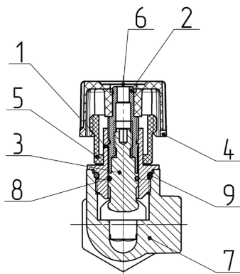
Рисунок 2 – Конструкция клапана
