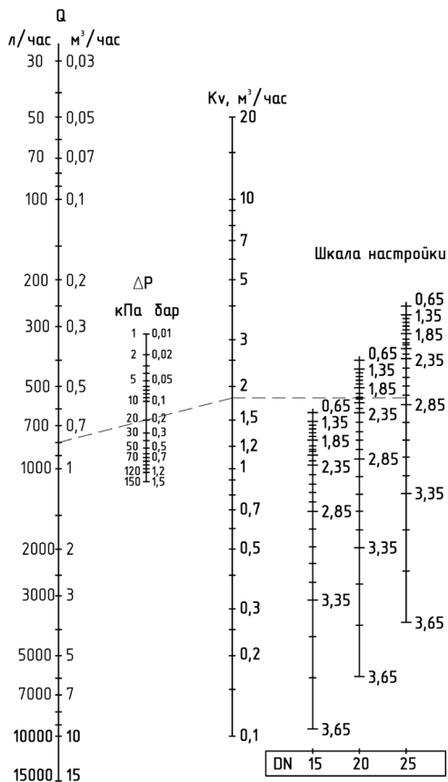
Рисунок 1. Номограмма подбор и настройка клапанов 2013
