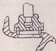
Рис. 2 Исполнение для т/ф 15кч16нж, остальное см. рис. 1
