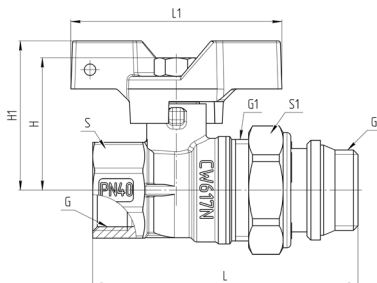
Рисунок 2 – Габаритные размеры крана.
