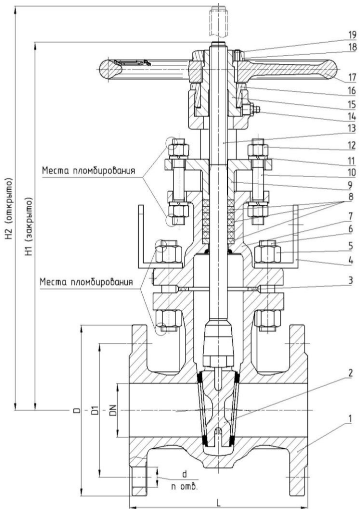
1–Корпус; 2–Клин; 3–Прокладка; 4–Кронштейн; 5–Гайка; 6–Штилька; 7–Крышка; 8–Набивка сальниковой камеры; 9–Сальник; 10–Штилька; 11–Шайба; 12–Гайка; 13–Шпиндель; 14–Масленка; 15–Втулка ходовая; 16–Втулка упорная; 17–Маховик; 18–Гайка; 19–Винт стопорный
