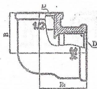
Рисунок 3. Угольник переходной
