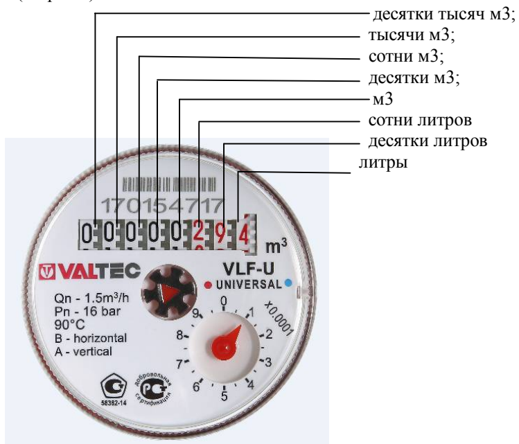
Рисунок 2. Табло счетчика
