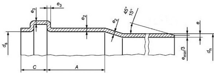
Рисунок 1. Размеры раструбов и трубных концов под уплотнительное кольцо.
