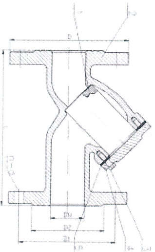
1 – сетка фильтрующая, 2 – корпус фильтра, 3 – болт, 4 – крышка фильтра, 5 – прокладка уплотнительная
