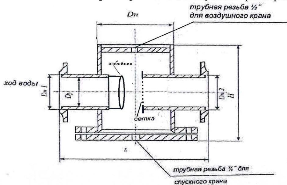
Фланцевое исполнение
