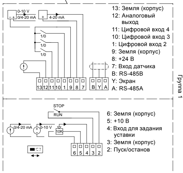
Рис. 4 Клеммы соединений, расширенный модуль ввода/вывода
