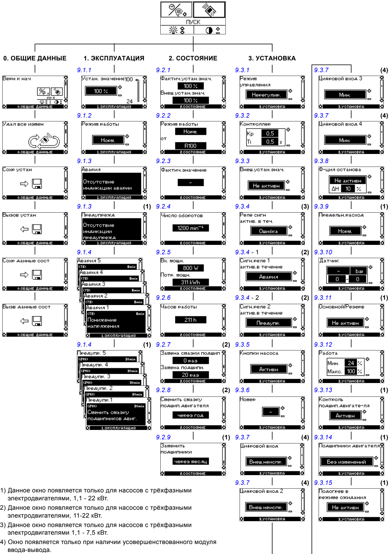
Рис. 23 Обзор меню
