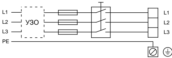
Рис. 2 Насос, подключенный к сети с сетевым выключателем, резервными плавкими предохранителями, дополнительной защитой и защитным заземлением
