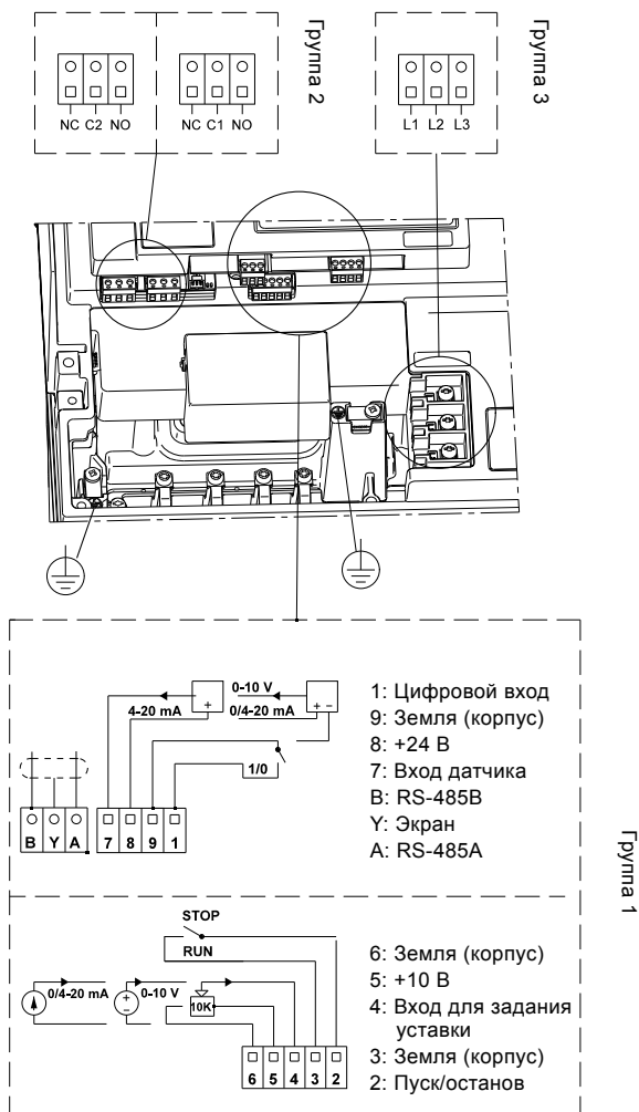
Рис. 5 Клеммы соединений, модуль ввода/вывода насоса
