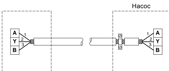
Рис. 12 Присоединение 3-жильного экранированного кабеля
