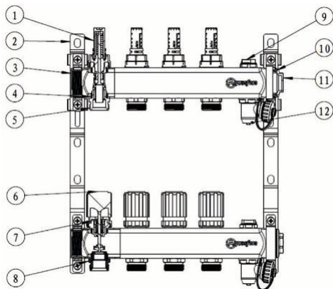
Описание коллекторной группы с расходомерами 9501
