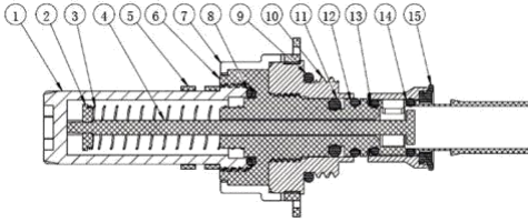
Конструкция и спецификация материалов расходомера коллектора 9501
