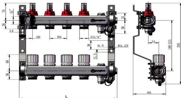
Габаритные и присоединительные размеры коллекторных групп 9501 Aquasfera
