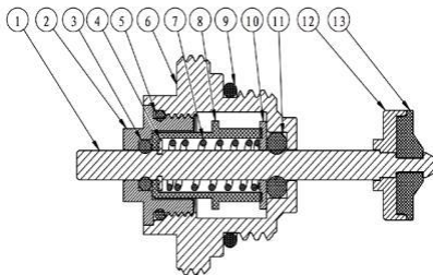
Конструкция и спецификация материалов расходомера коллектора 9501
