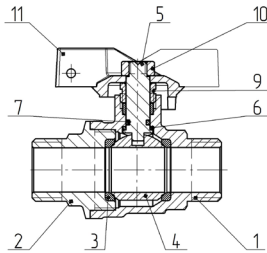
Рисунок 1 – Конструкция шарового крана
