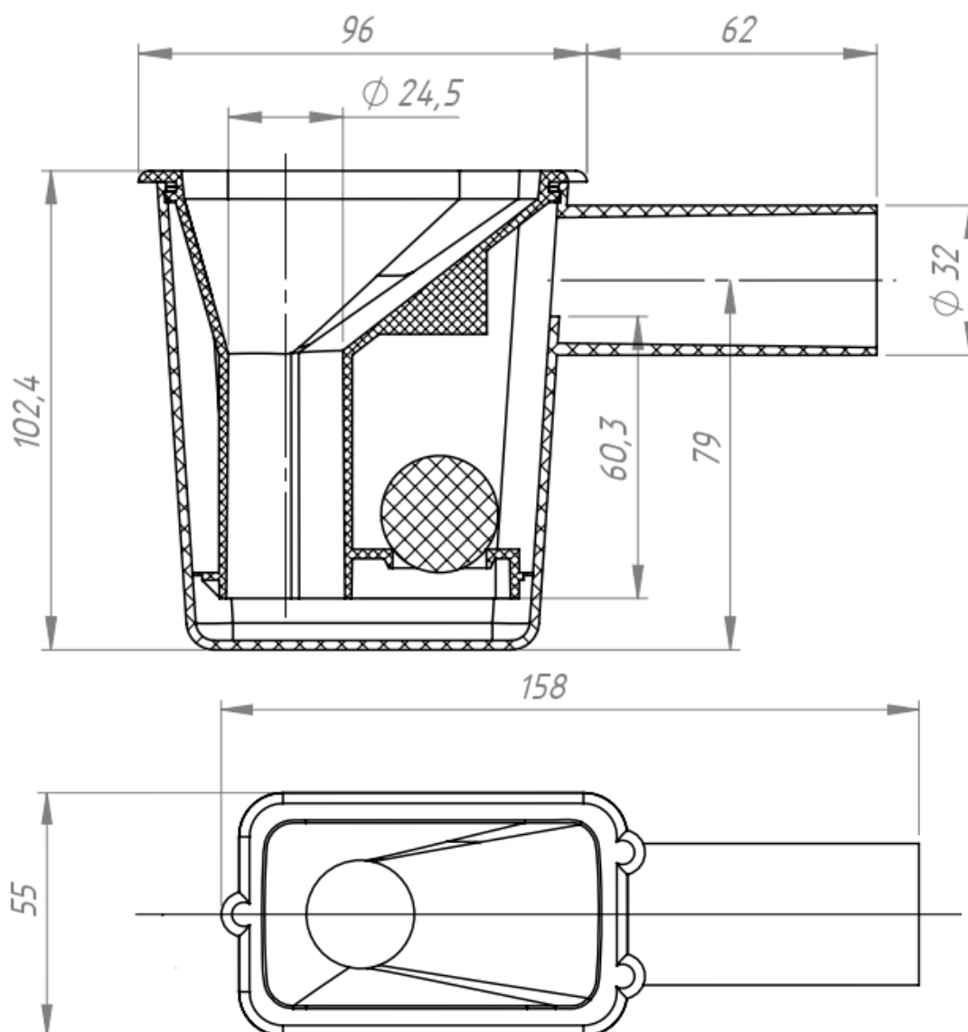
Рис. 1. Схема капельной воронки
