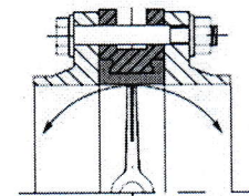
Рис. 3 (правильно)
