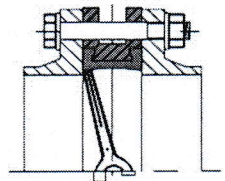
Рис. 1 (неправильно)
