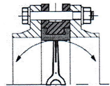
Рис. 2 (неправильно)
