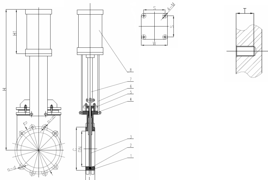
Рис. 1. Габаритные и присоединительные размеры шиберной задвижки.
