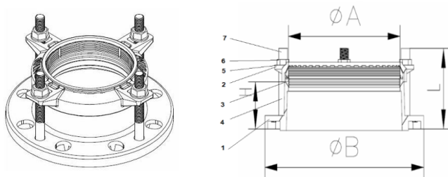
Рис.4. Муфта/адаптер ПФРК-Е
