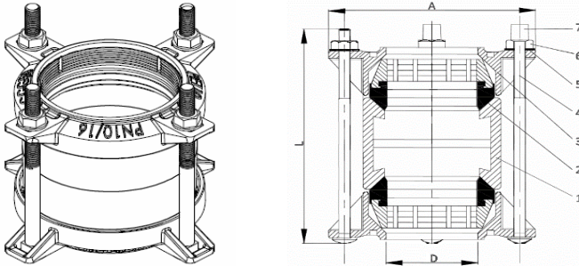
Рис.2. Муфта ДРК-Е
