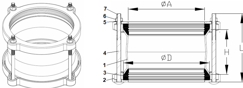
Рис.1. Муфта ДРК
