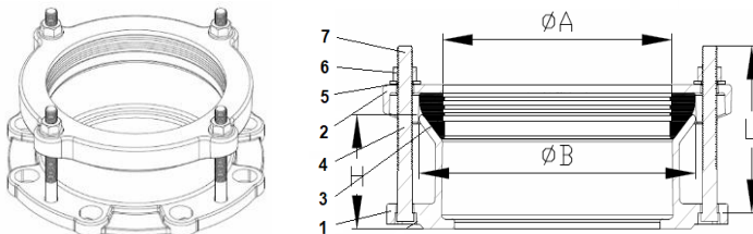
Рис.3. Муфта/адаптер ПФРК
