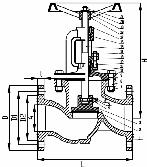
Рис. 1. Клапан запорный чугунный фланцевый.
