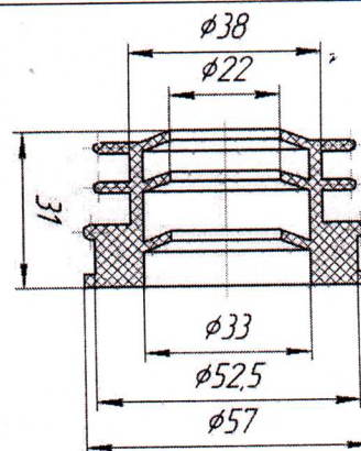
Манжета переходная D 50x25 трех лепестковая
