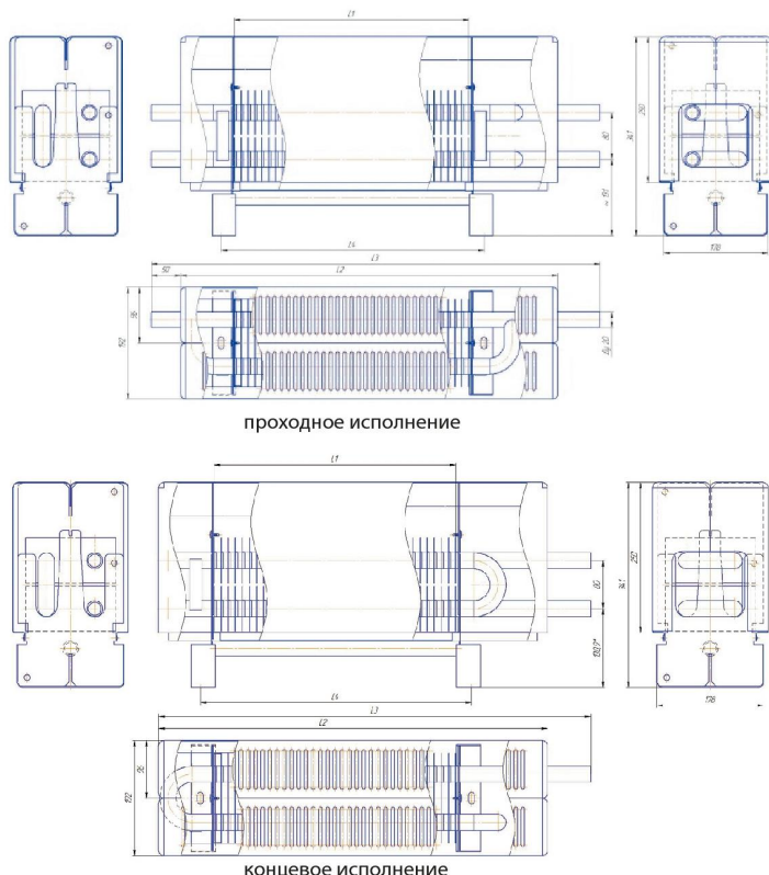
Рис. 9 Конвектор ТЗПО «КПНК» (концевой)
