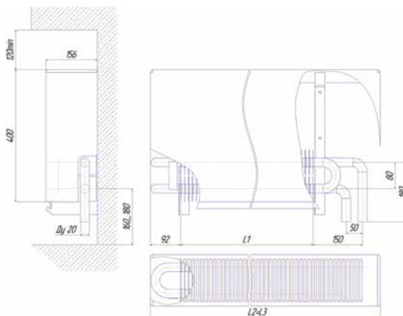
концевое исполнение
