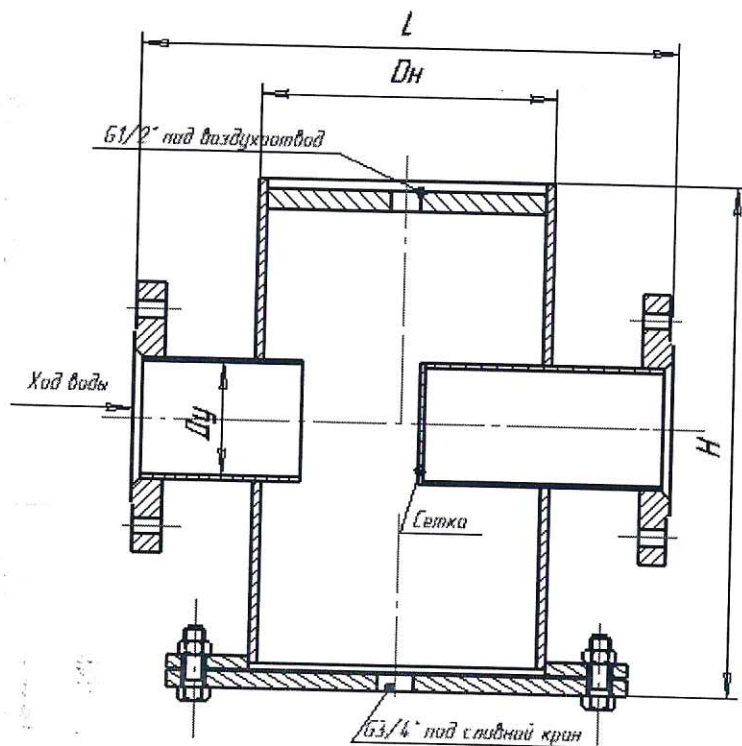
2 Исполнение фланцевое
