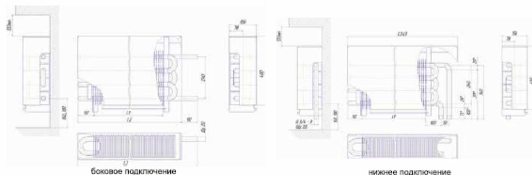
Рис. 8. Конвектор ТЗПО «Универсал Супер»
