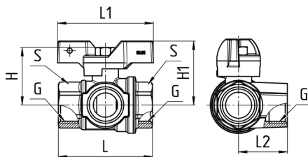
Рисунок 2 – Габаритные размеры крана.
