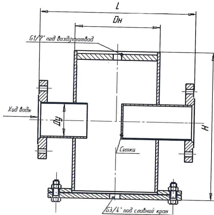
2 Исполнение фланцевое
