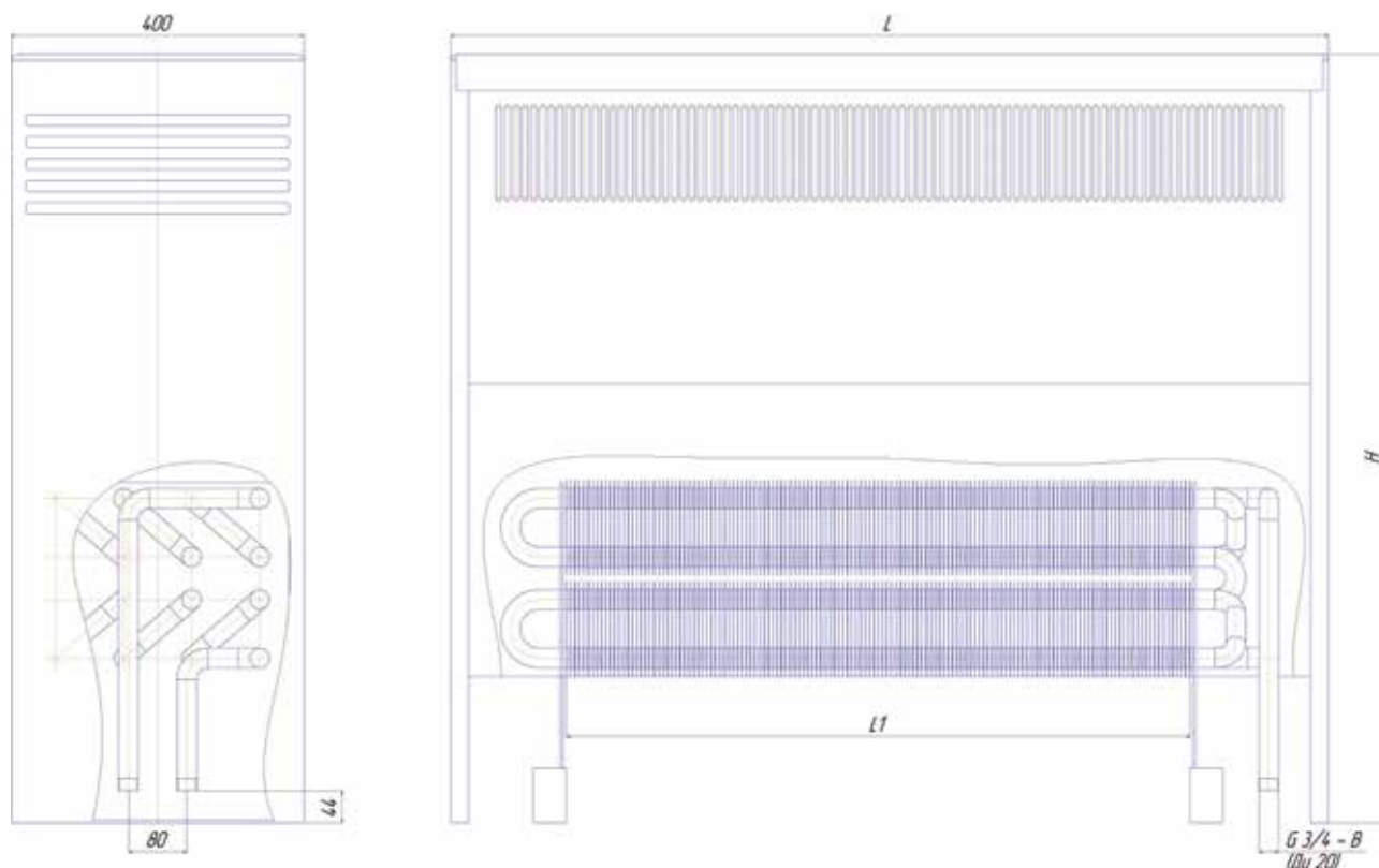
Рис. 10 Конвектор ТЗПО «КПВК»
