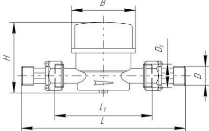
Рисунок 1 – схематическое изображение счетчика.
