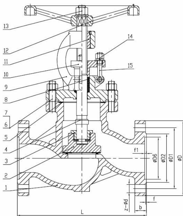
Рис.1 Клапан запорный фланцевый 15нж22нж.
