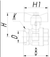
Основные размеры
