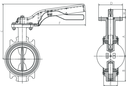
R59WY004 – 030, R59FLY004 – 030
