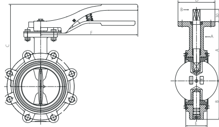
R59WX004 – 030, R59FLX004 – 030
