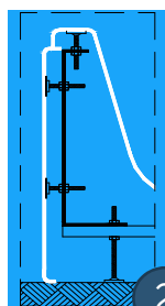
МАГНИТНЫЕ ОПОРЫ ФИКСИРУЮТСЯ К ПАНЕЛИ
