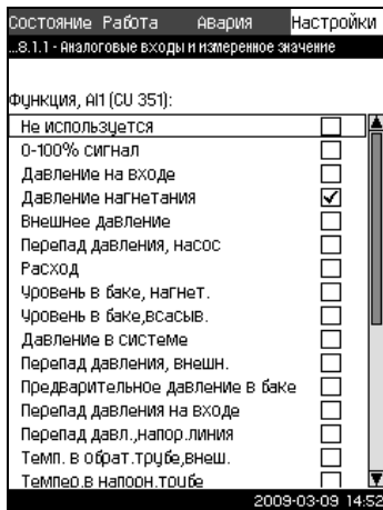
Рис. 74 Аналоговые входы и измеренное значение
