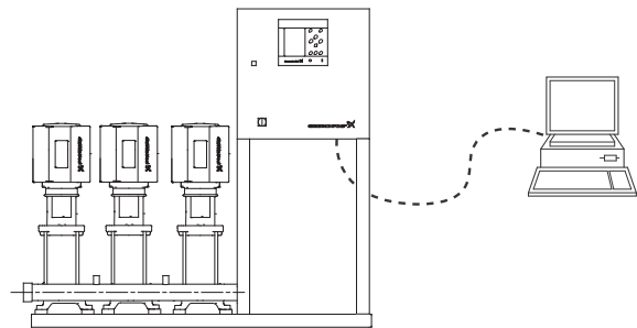
Рис. 23 Установка повышения давления с внешним контроллером (разомкнутый контур)
