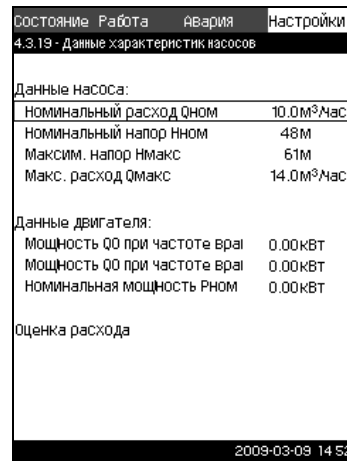
Рис. 81 Данные характеристик насосов
