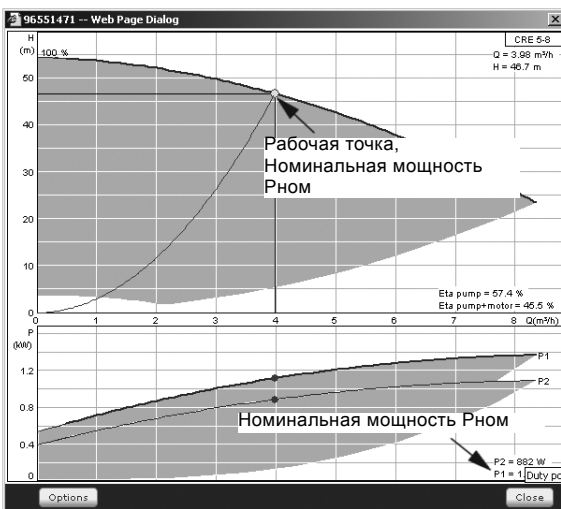
Рис. 85 Значение номинальной мощности Pном (WebCAPS)
