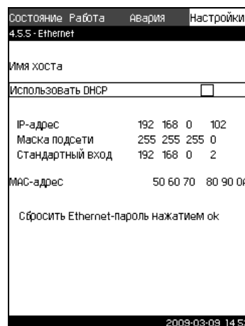
Рис. 111 Пример настройки Ethernet
