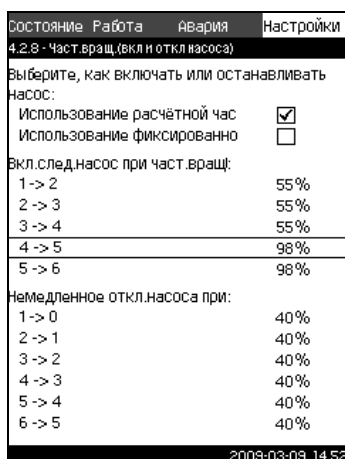
Рис. 57 Расчётная частота вращения, при которой насос включается или отключается
