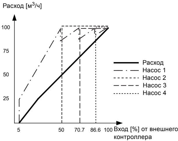
Рис. 26 Регулировочная характеристика для Hydro MPC-F в разомкнутом контуре
