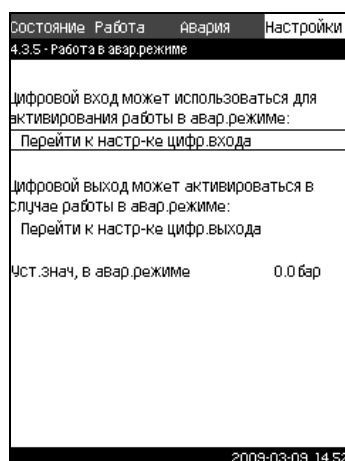
Рис. 69 Работа в аварийном режиме
