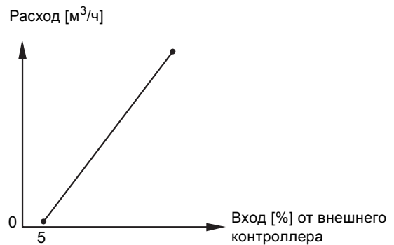
Рис. 24 Регулировочная характеристика для разомкнутого контура
