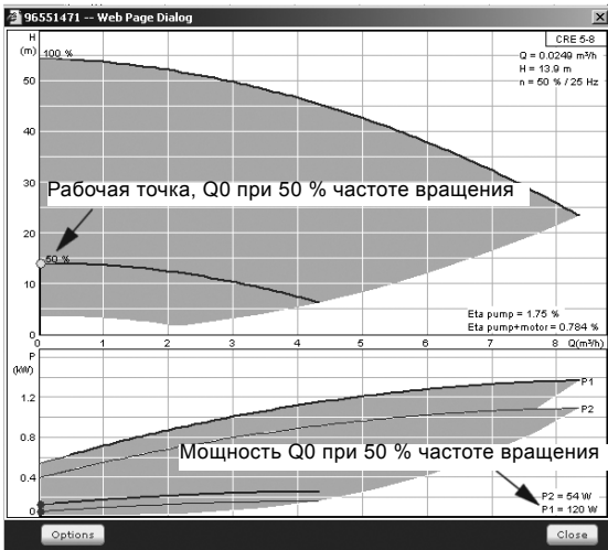
Рис. 84 Показание мощности Q0 при 50 % частоте вращения (WebCAPS)
