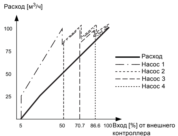
Рис. 25 Регулировочная характеристика для Hydro MPC-E в разомкнутом контуре
