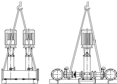
Fig. 4 Правильный подъём Hydro MPC XL
