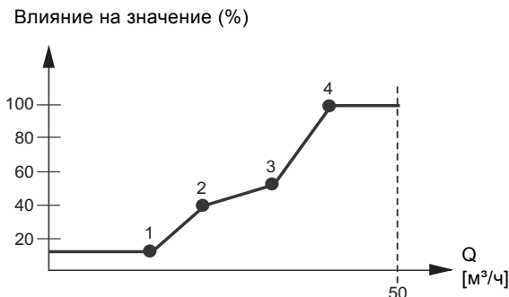
Рис. 41 Соотношение между влиянием на установленное значение и расходом
