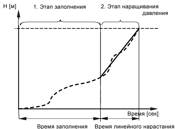
Рис. 68 Этапы заполнения и нарастания давления
