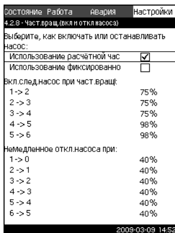
Рис. 58 Фиксированная частота вращения для пуска и останова насоса
