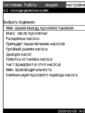
Рис. 49 Каскадное управление насосами
