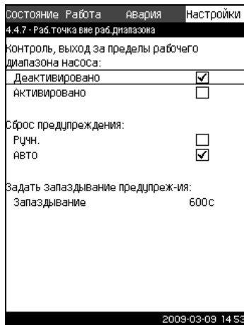
Рис. 98 Выход рабочей точки насоса за пределы рабочего диапазона
