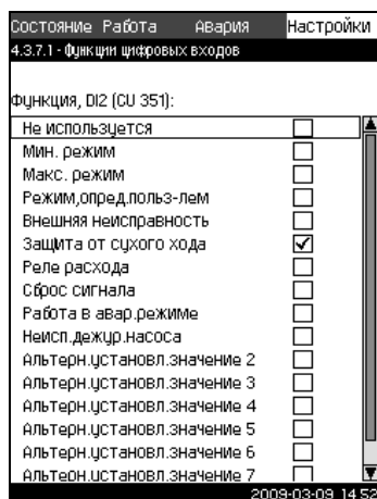
Рис. 71 Функции цифровых входов
