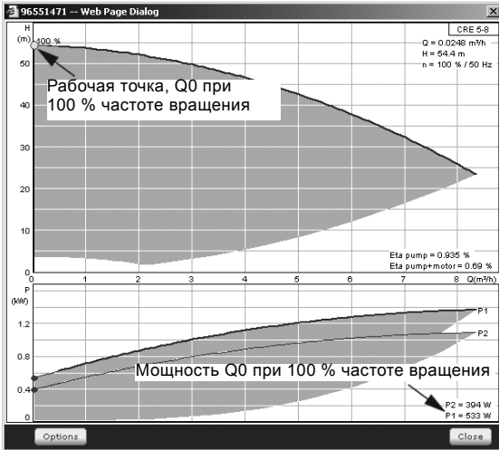
Рис. 83 Показание мощности Q0 при 100 % частоте вращения (WebCAPS)
