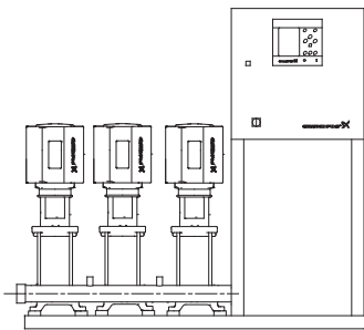
Рис. 21 Установка, регулируемая встроенным ПИ контроллером (замкнутый контур)
