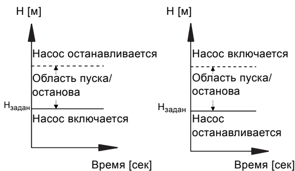
Рис. 48 Нормальное и обратное управление
