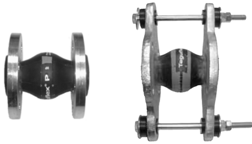
Рис. 6 Вибровставки с резиновыми прокладками без ограничительных стяжек и с ними
