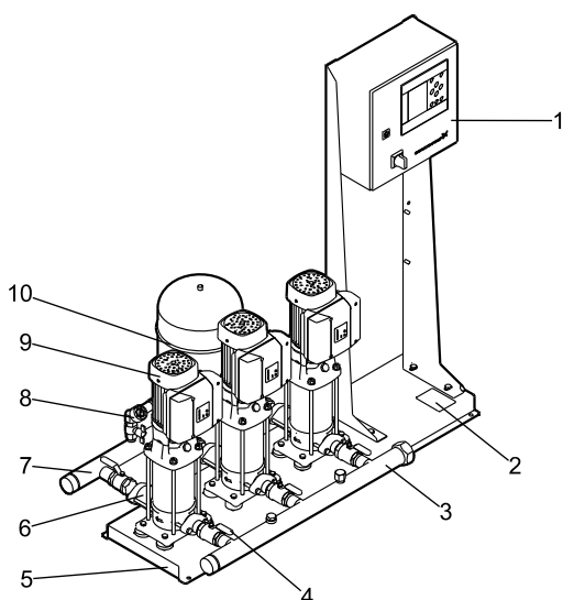
Рис. 1 Система повышения давления Hydro MPC
