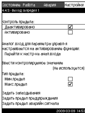
Рис. 97 Выход за предел 1
