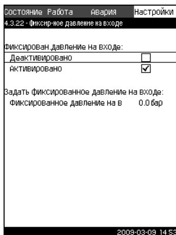
Рис. 87 Фиксированное давление на входе
