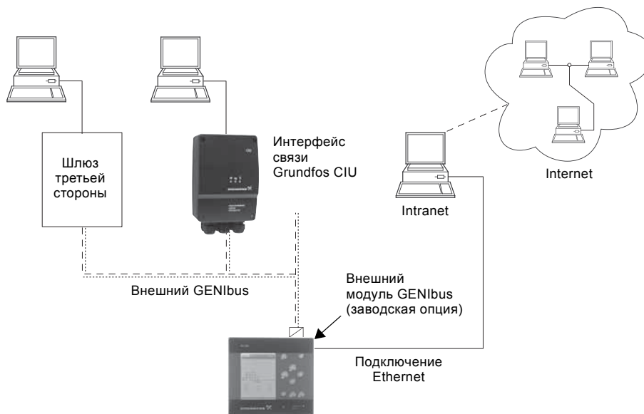
Рис. 110 Передача данных через внешнее соединение GENIbus и локальную сеть
