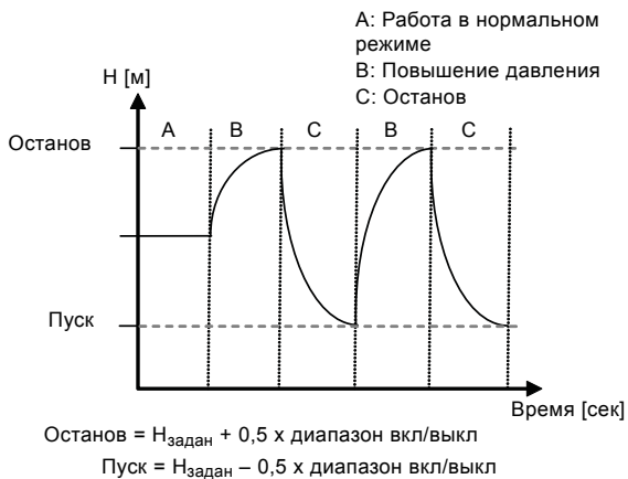
Рис. 64 Работа в режиме включения/выключения
