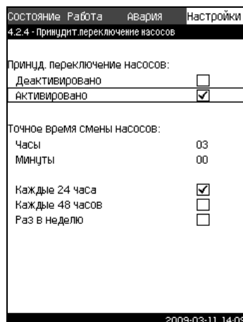
Рис. 53 Принудительное переключение насосов
