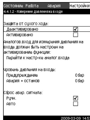
Рис. 92 Защита от "сухого хода" с помощью датчика давления
