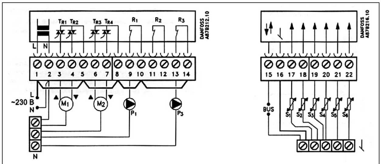
Рис. 41. Схемы электрических соединений на 230 В к рис.26-29.
