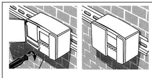
Рис. 54б. Установка корпуса на DIN - рейке.
