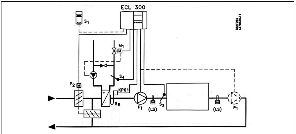
Рис. 4. Схема применения - 2.
