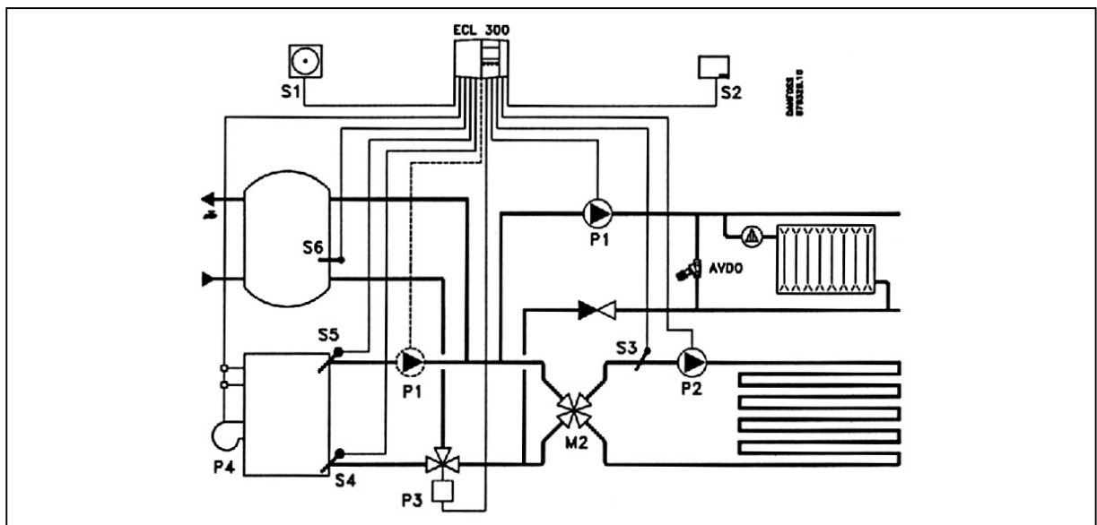
Рис. 23. Схема применения - 1.
