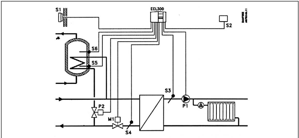
Рис. 22. Схема применения - 5.
