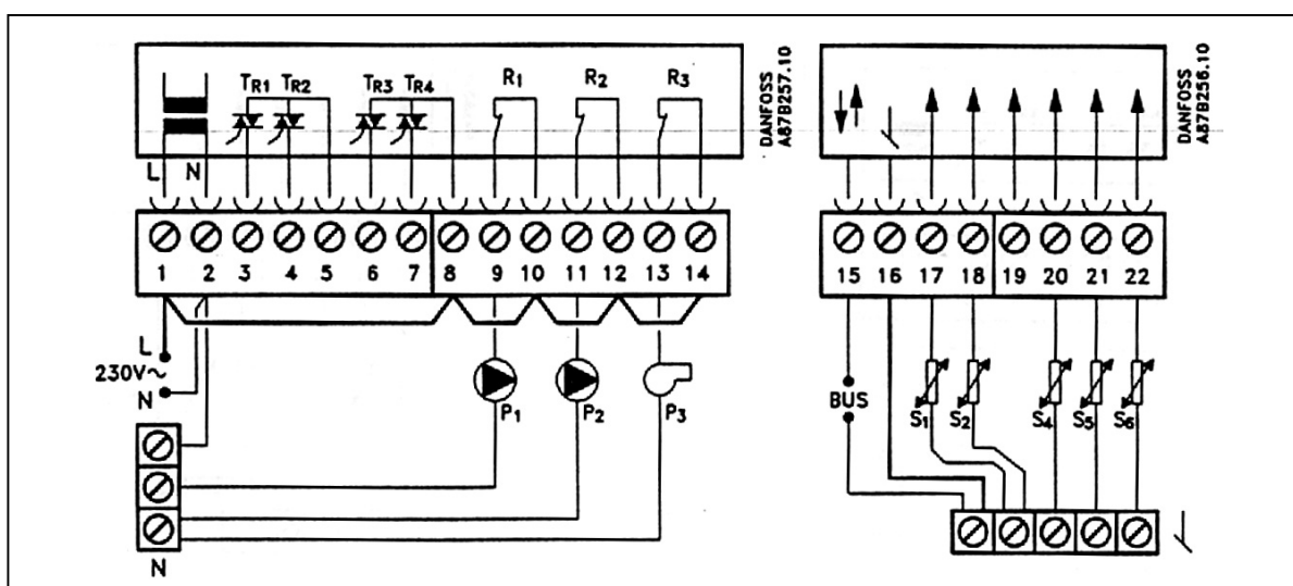
Рис. 37. Схемы электрических соединений на 230 В к рис.11-13.
