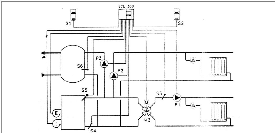
Рис. 32. Схема применения - 1.
