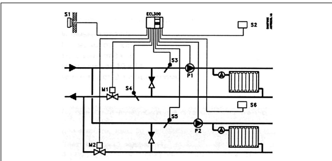
Рис. 26. Схема применения - 1.
