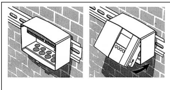
Рис. 54а. Установка корпуса на DIN - рейке.
