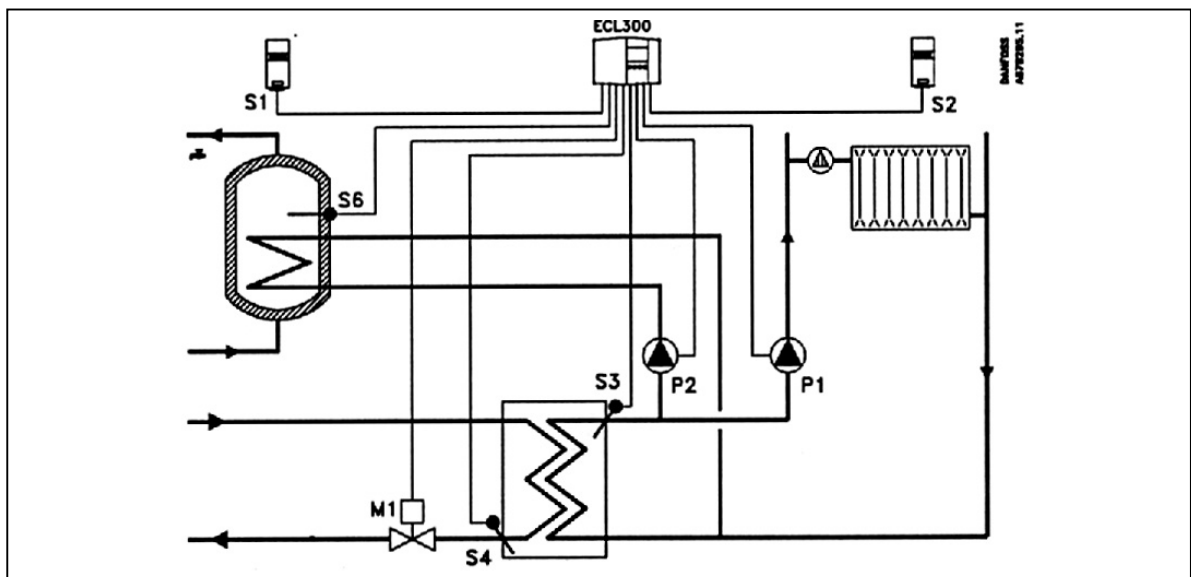
Рис. 14. Схема применения - 1.
