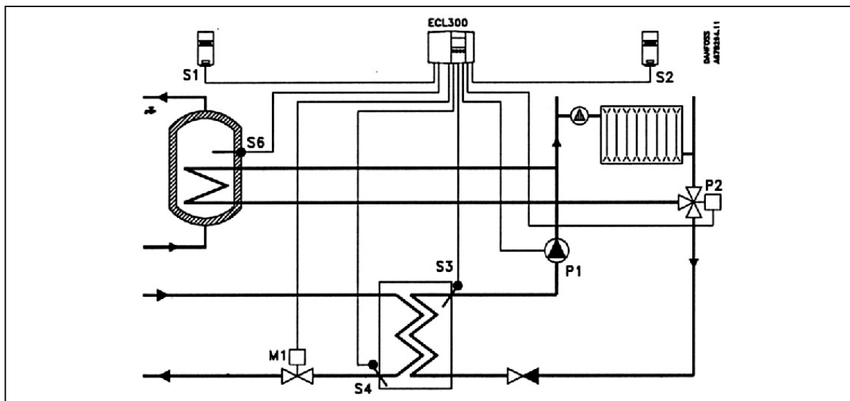
Рис. 14. Схема применения - 1.
