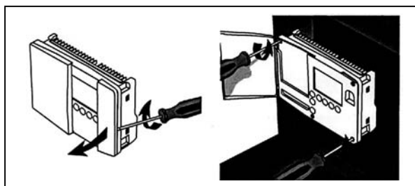
Рис. 55а. Установка корпуса в шкафу управления.
