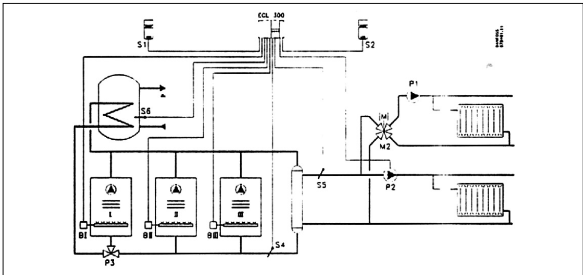
Рис. 34. Схема применения – 2б.
