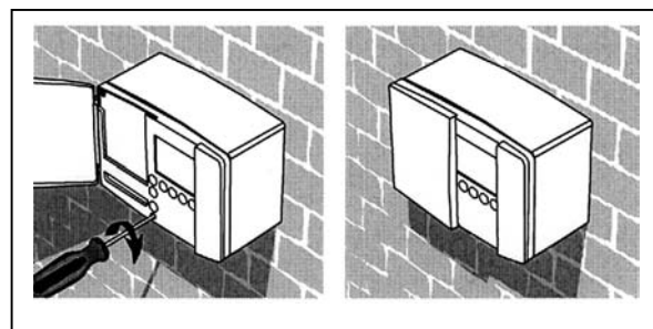
Рис. 53б. Установка корпуса на стену.
