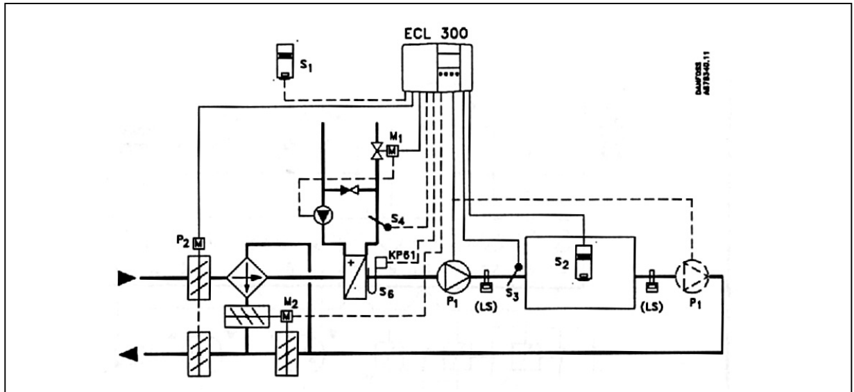
Рис. 8. Схема применения - 6.
