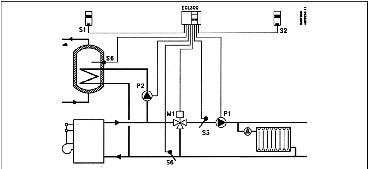
Рис. 17. Схема применения - 4.
