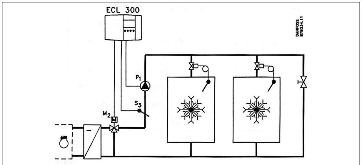
Рис. 9. Схема применения - 7.
