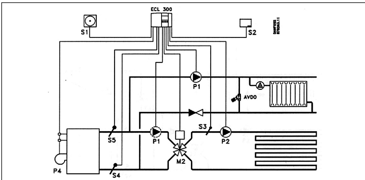
Рис. 25. Схема применения - 3.
