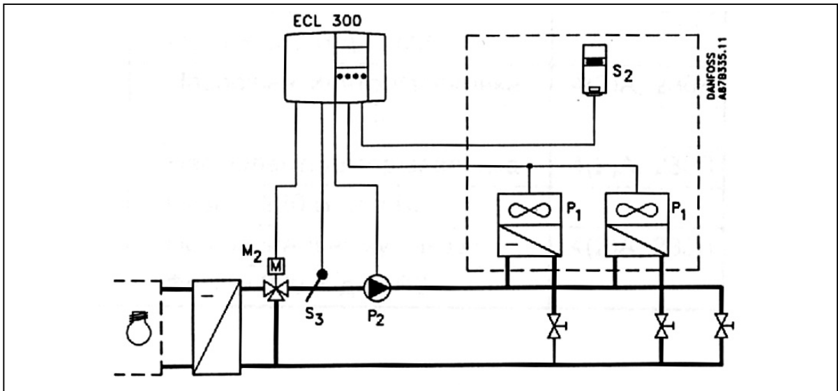
Рис. 10. Схема применения - 8.
