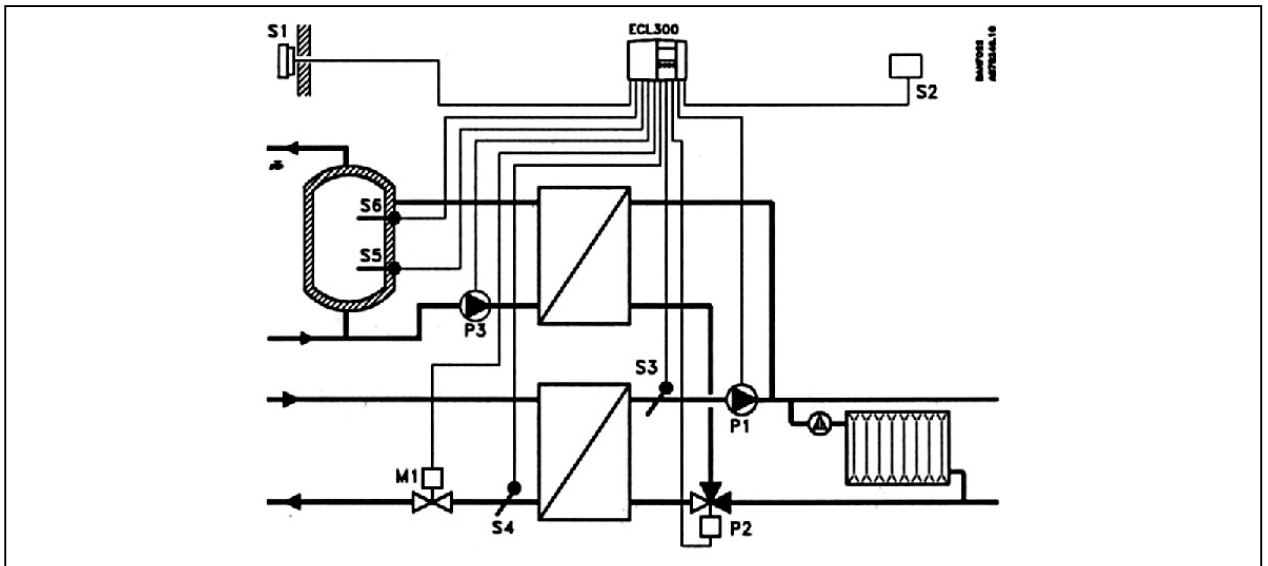
Рис. 19. Схема применения - 2.
