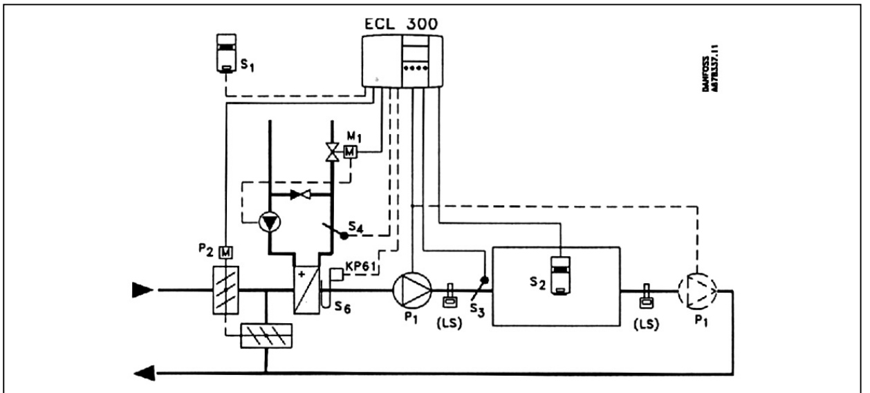
Рис. 5. Схема применения - 3.
