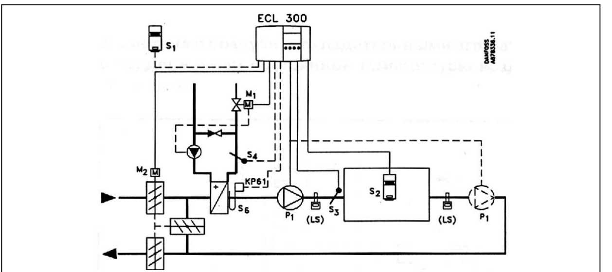
Рис. 5. Схема применения - 3.
