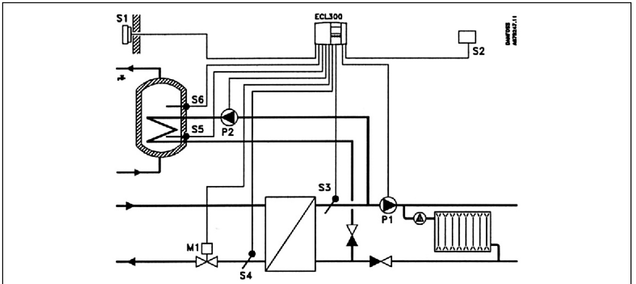
Рис. 20. Схема применения - 3.
