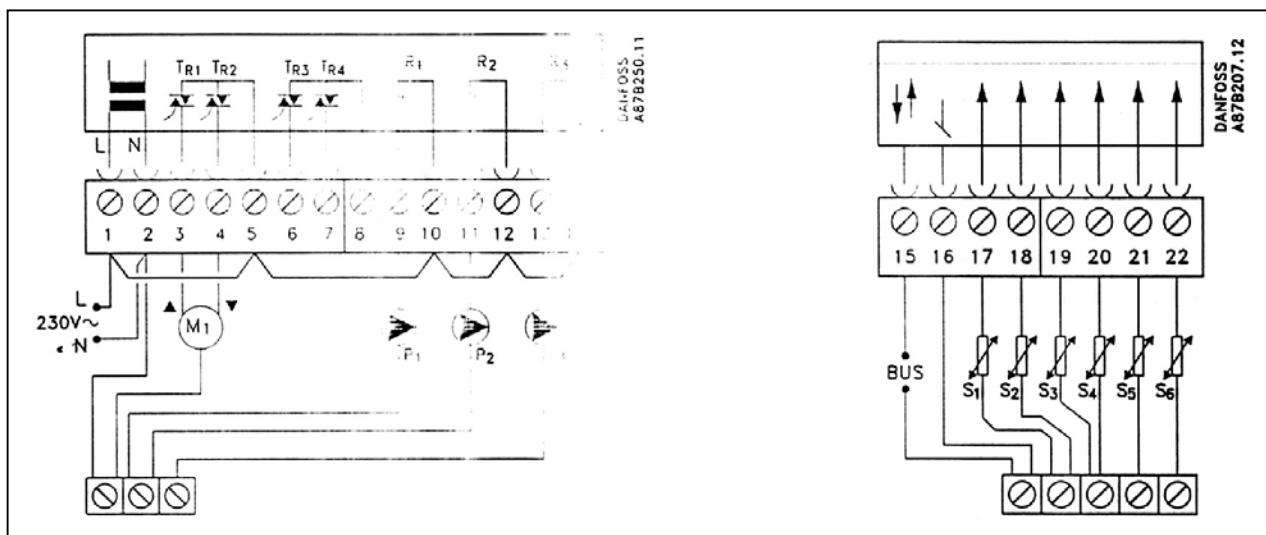
Рис. 39. Схемы электрических соединений на 230 В к рис.18-22.
