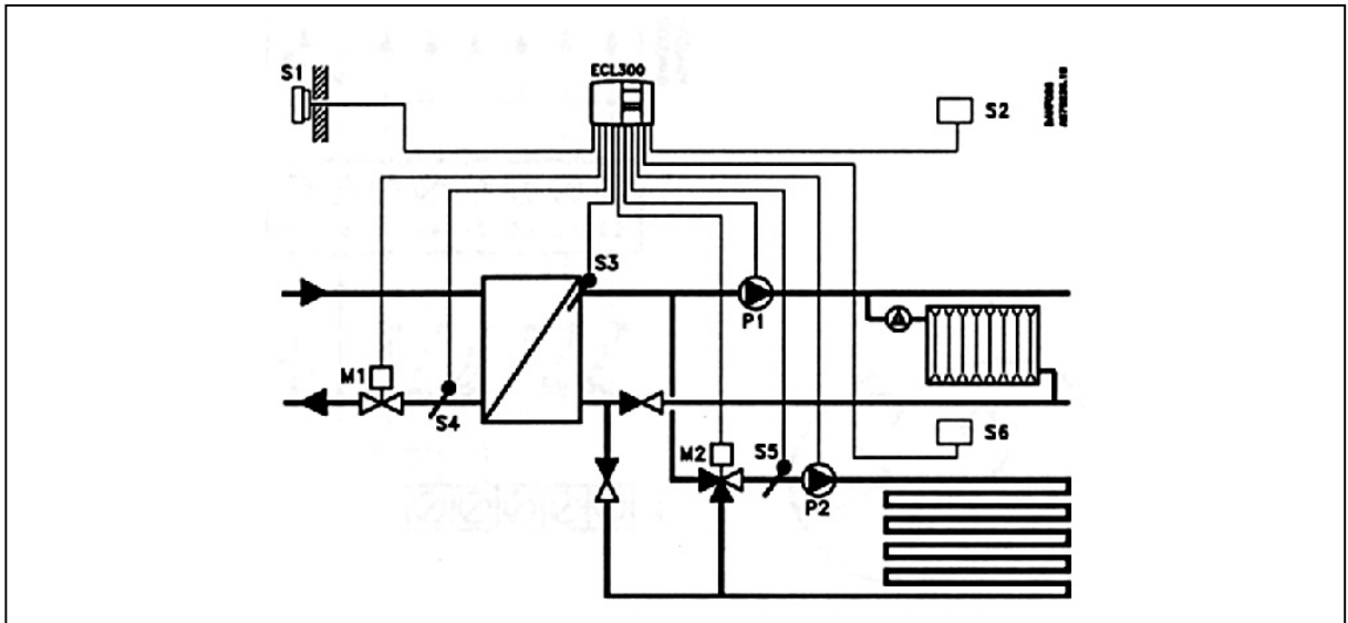
Рис. 28. Схема применения - 3.
