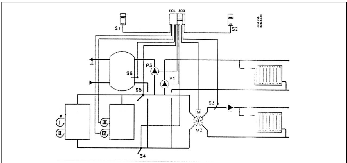
Рис. 35. Схема применения – 3.
