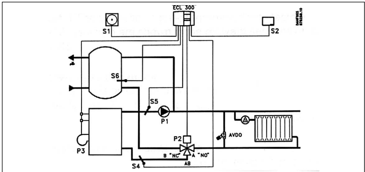
Рис. 11. Схема применения - 1.
