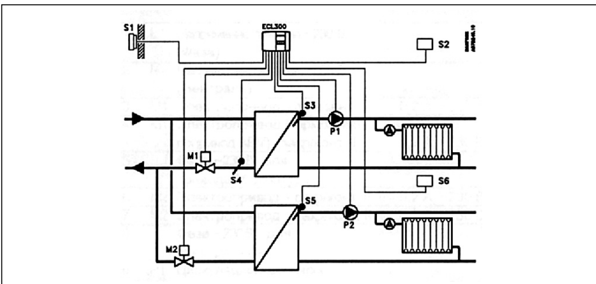
Рис. 26. Схема применения - 1.
