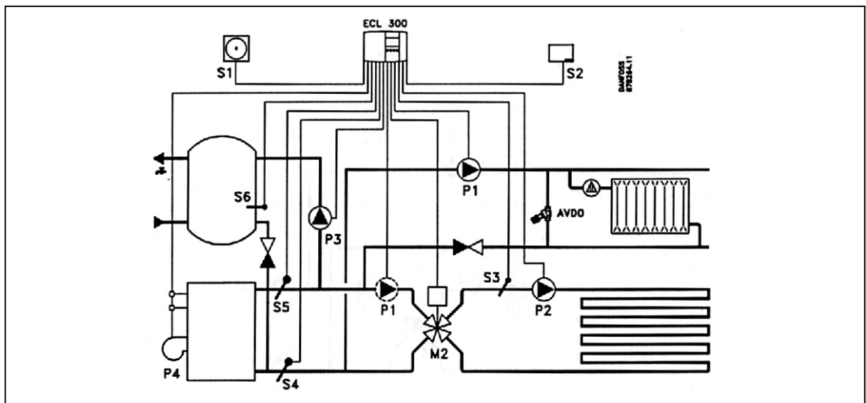
Рис. 23. Схема применения - 1.
