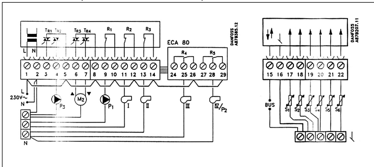
Рис. 44. Схемы электрических соединений на 230 В к рис.33, 34.
