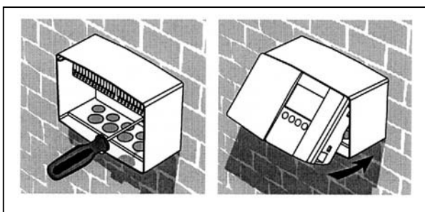
Рис. 53а. Установка корпуса на стену.
