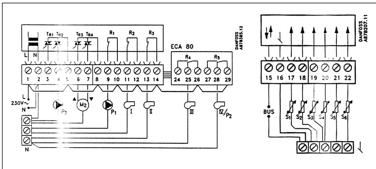
Рис. 45. Схемы электрических соединений на 230 В к рис.35.
