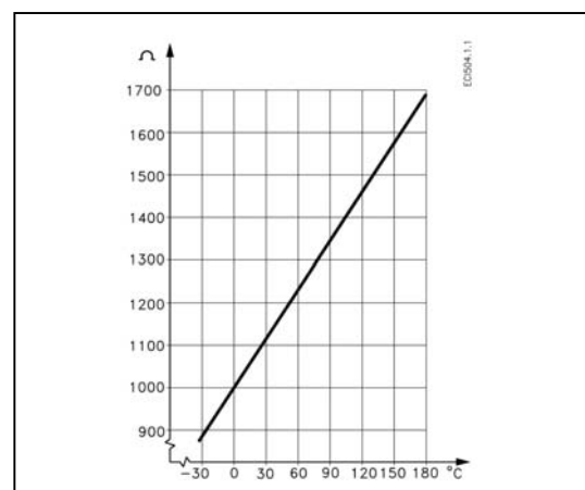
Рис. 58. График изменения сопротивления.
