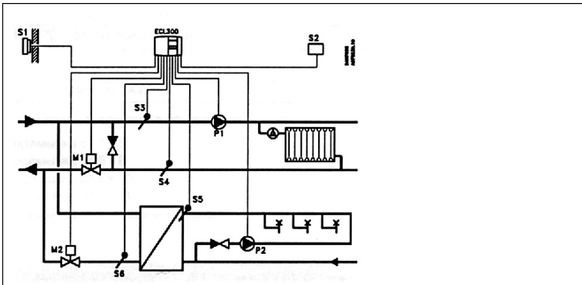
Рис. 31. Схема применения - 2.
