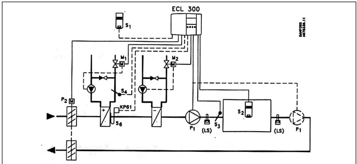
Рис. 7. Схема применения - 5.
