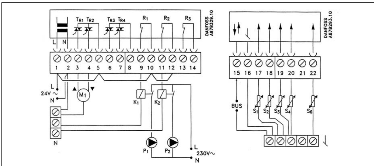
Рис. 48. Схемы электрических соединений на 24 В к рис.14-17.
