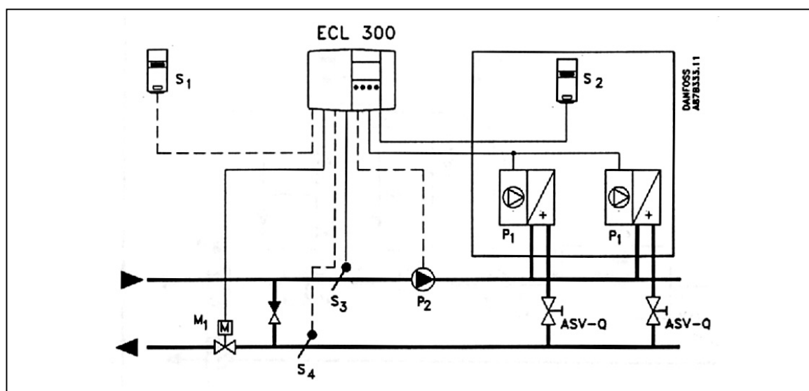
Рис. 3. Схема применения - 1.
