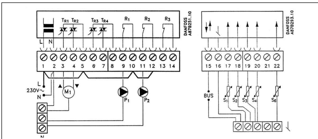
Рис. 38. Схемы электрических соединений на 230 В к рис.14-17.
