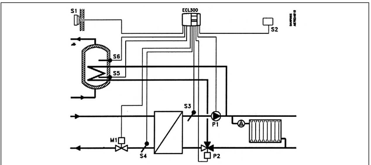
Рис. 21. Схема применения - 4.
