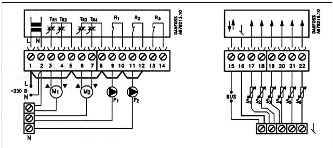
Рис. 42. Схемы электрических соединений на 230 В к рис.30,31.
