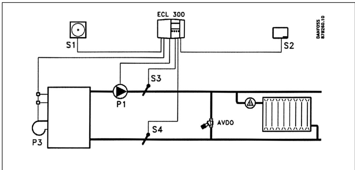
Рис. 13. Схема применения - 3.
