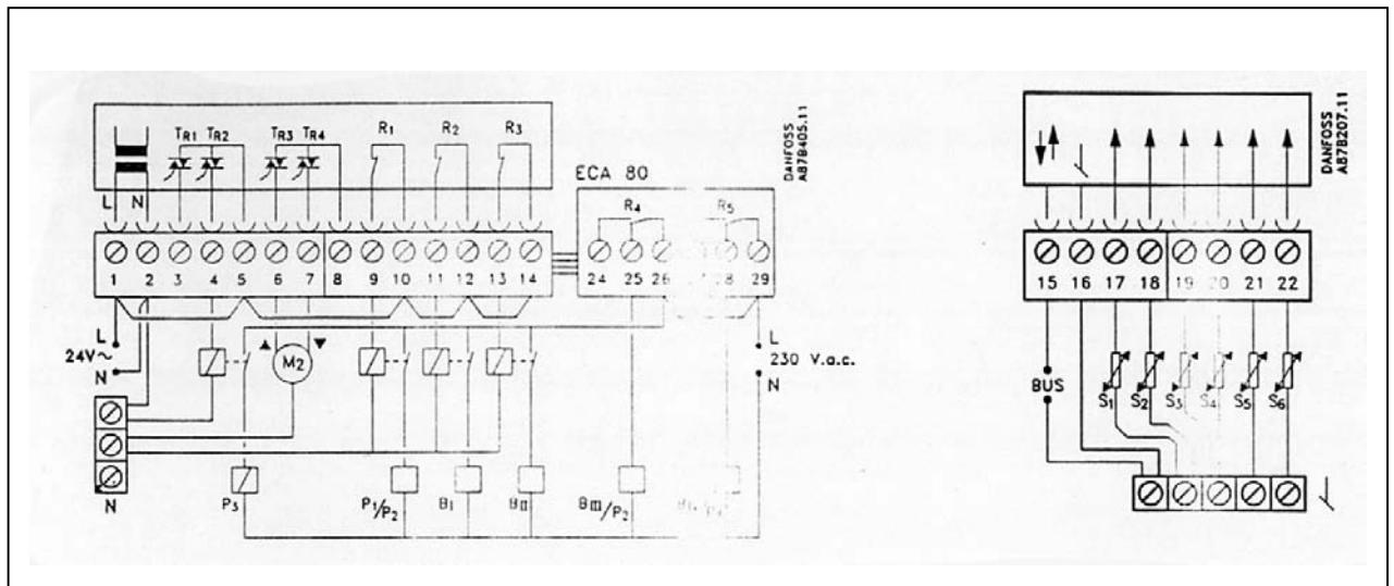
Рис. 51. Схемы электрических соединений на 24 В к рис.32-35.
