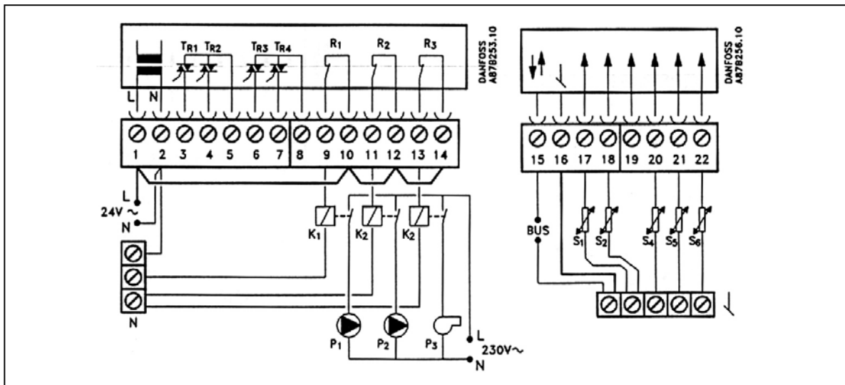
Рис. 47. Схемы электрических соединений на 24 В к рис.11-13.
