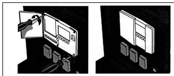
Рис. 55б. Установка корпуса в шкафу управления.
