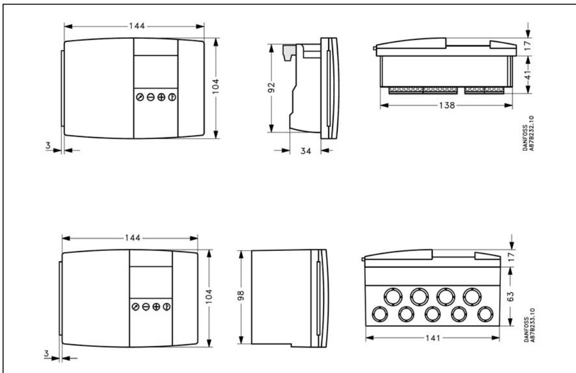
Рис. 56. Габаритные и присоединительные размеры электронного регулятора ECL 300.
