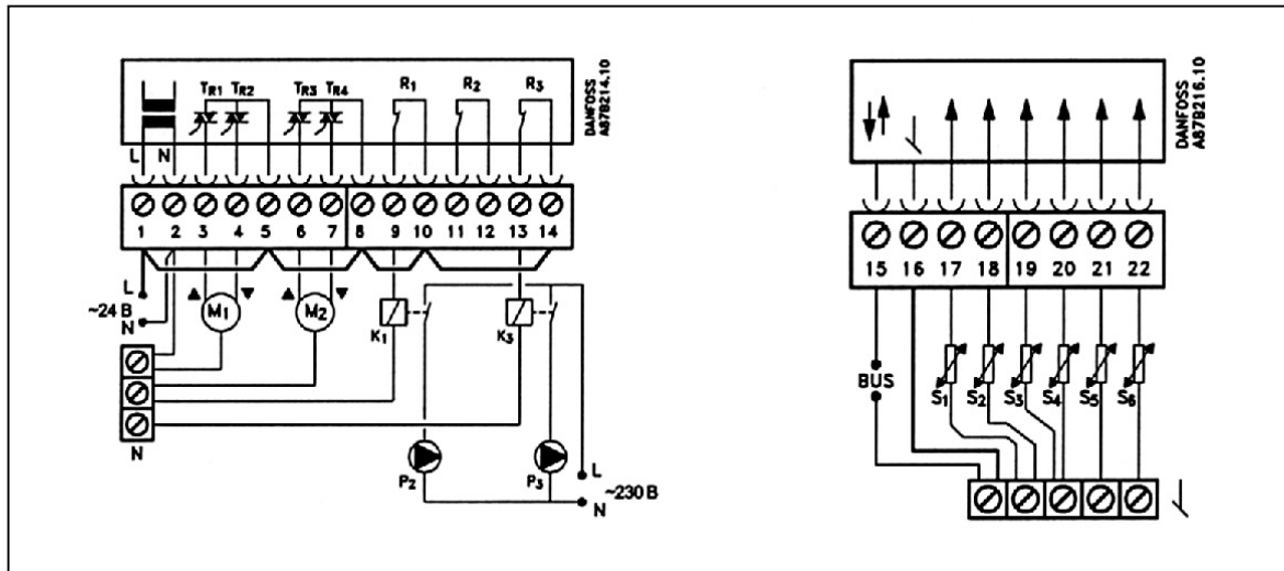
Рис. 50. Схемы электрических соединений на 24 В к рис.30,31.
