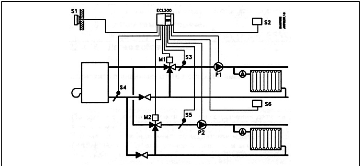
Рис. 29. Схема применения - 4.
