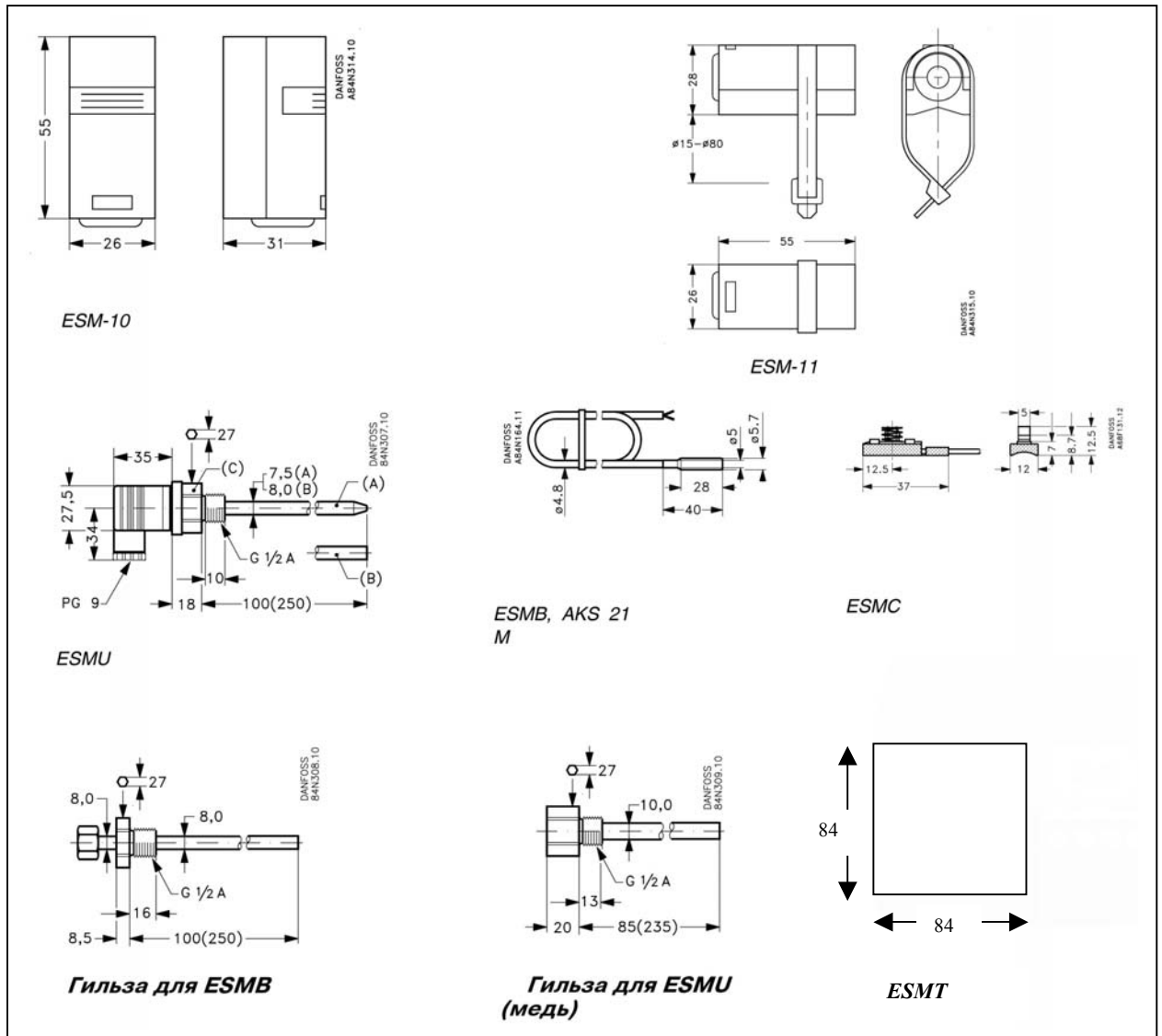
Рис. 59. Габаритные и присоединительные размеры датчиков температуры.
