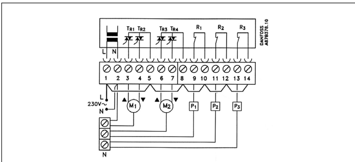
Рис. 36. Схемы электрических соединений на 230 В к рис.3-10.
