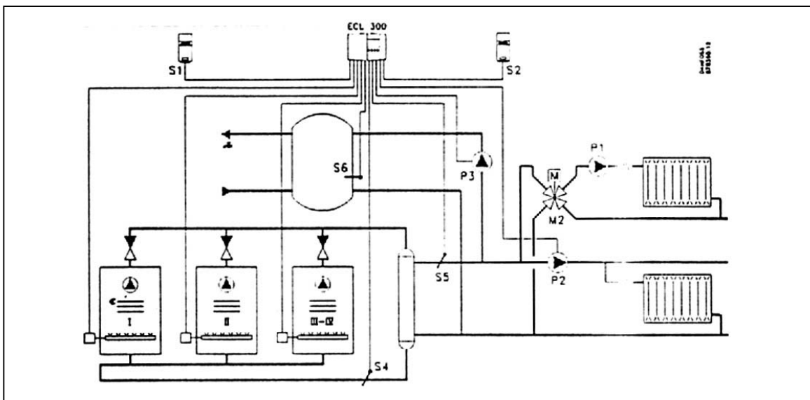
Рис. 32. Схема применения - 1.
