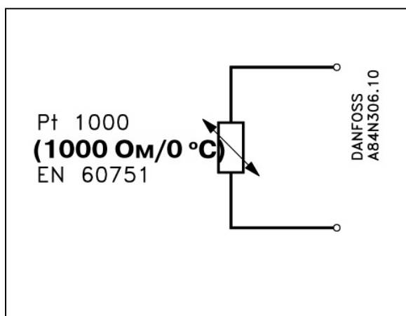
Рис. 57. Схемы электрического соединения датчика температуры.
