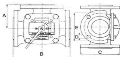
Тип F с фланцевыми соединениями
