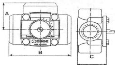
Тип G с винтовыми соединениями
