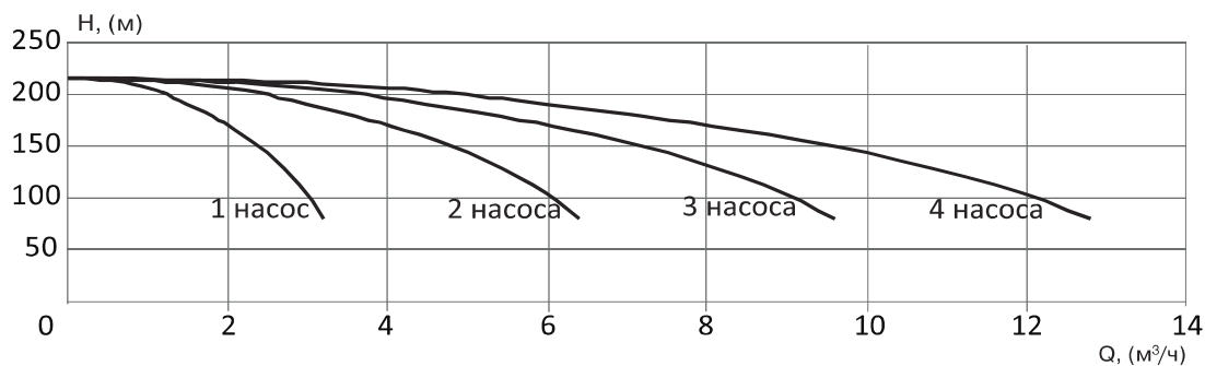
УНВ DPV 2/28 2,2 кВт
