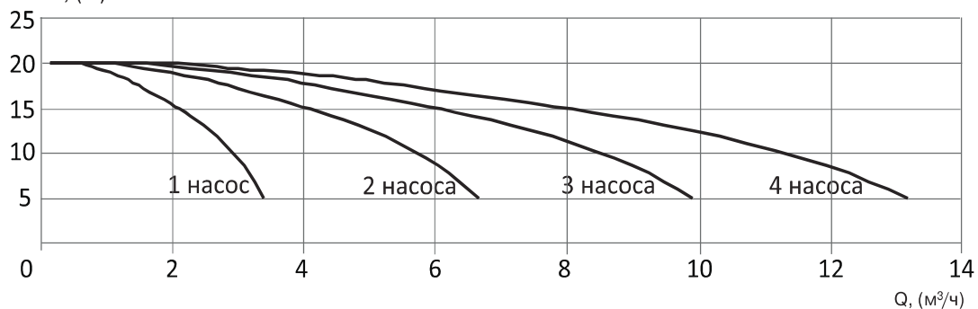
УНВ DPV 2/3 0,37 кВт H, (м)
