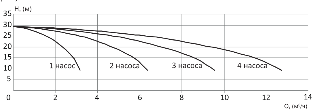
УНВ DPV 2/4 0,37 кВт H, (м)
