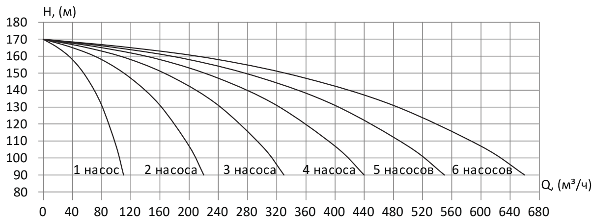
УНВ DPV 85/6-1 45,0 кВт
