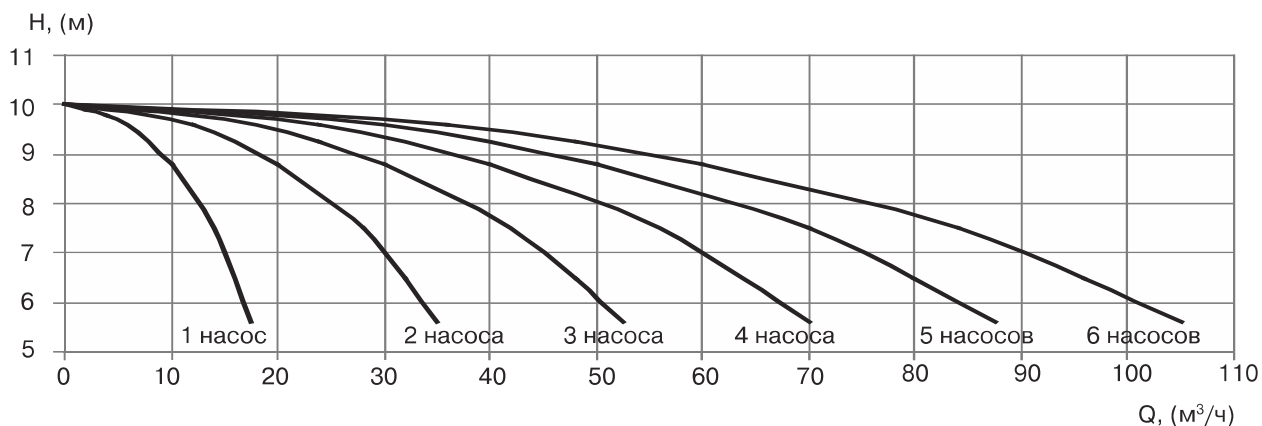
УНВ DPV 25/3 1,1 кВт H, (м)
