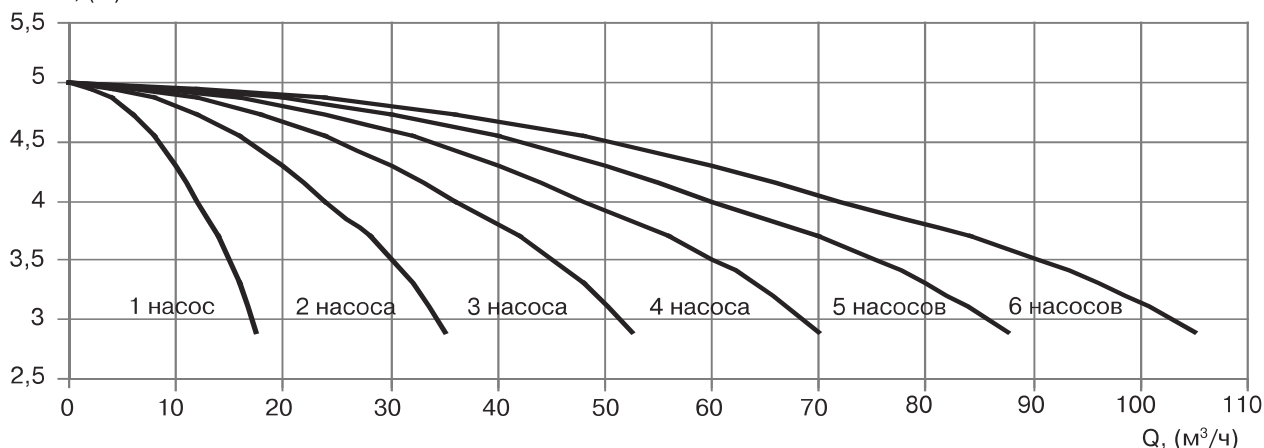
УНВ DPV 25/1 1,1 кВт H, (м)
