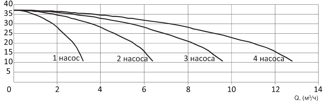
УНВ DPV 2/5 0,37 кВт H, (м)
