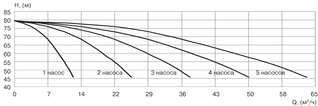
УНВ DPV 10/8 3,0 кВт
