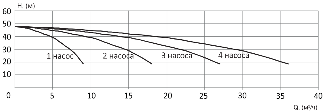
УНВ DPV 6/5 1,1 кВт
