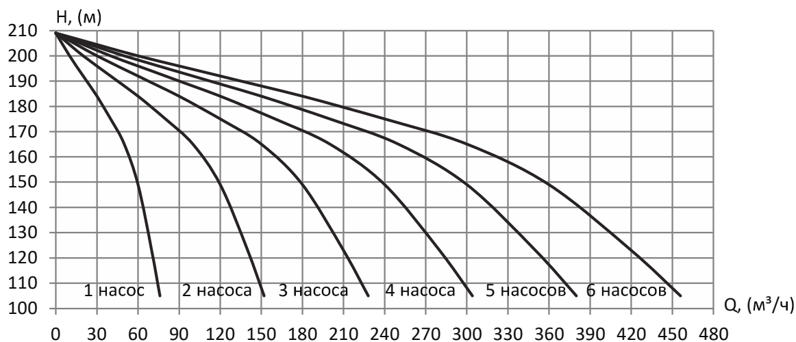
УНВ DPV 60/8-2 37,0 кВт
