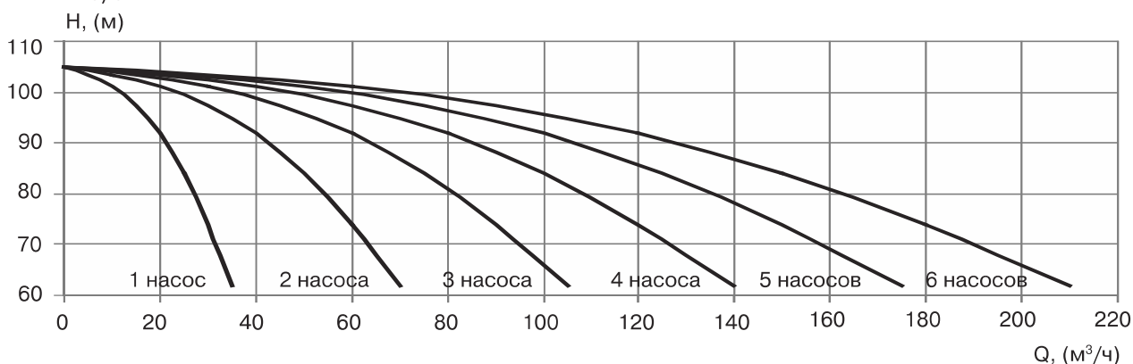
УНВ DPV 25/5 11 кВт
