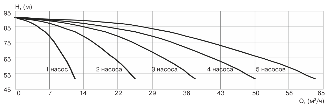
УНВ DPV 10/8 3,0 кВт
