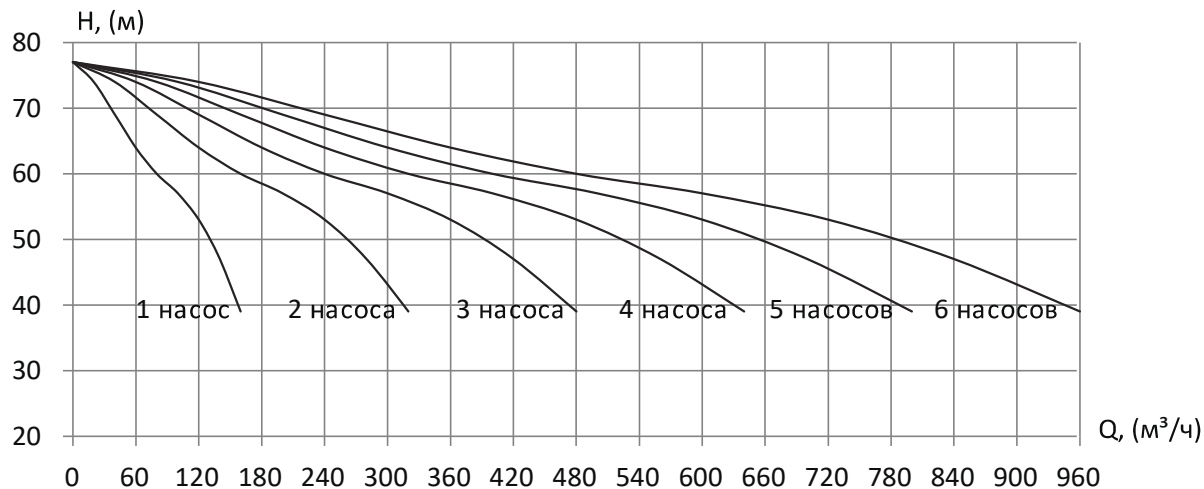
УНВ DPV 125/2 30,0 кВт
