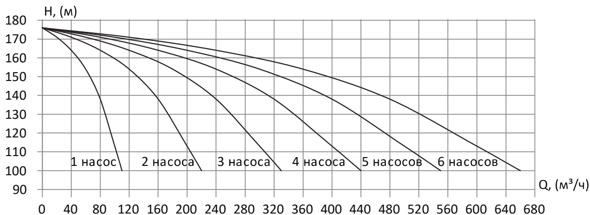
УНВ DPV 85/6 45,0 кВт
