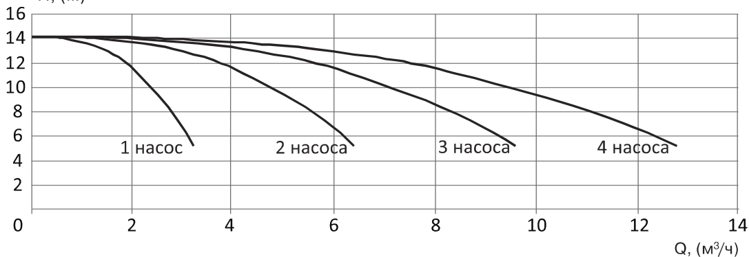
УНВ DPV 2/3 0,37 кВт H, (м)
