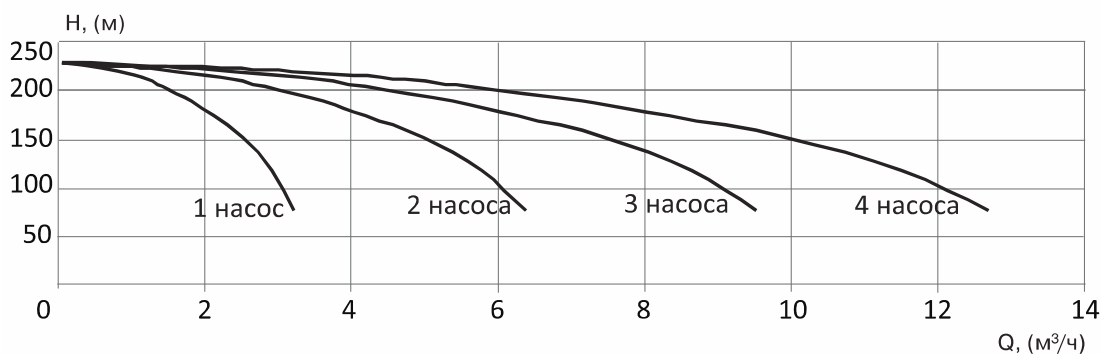
УНВ DPV 2/30 2,2 кВт
