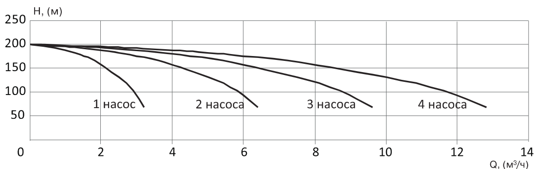
УНВ DPV 2/26 2,2 кВт
