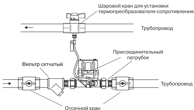
Рис. 9. Пример монтажа теплосчетчика
