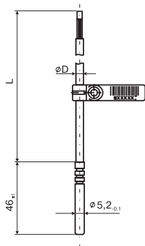
Рис. 1. Температурный датчик типа Pt 500
