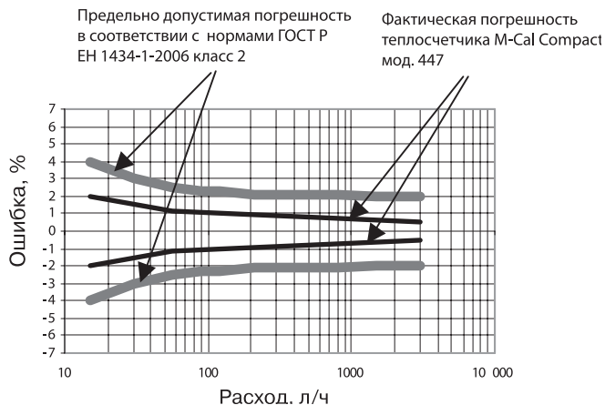
Рис. 2. Метрологические характеристики теплосчетчиков
