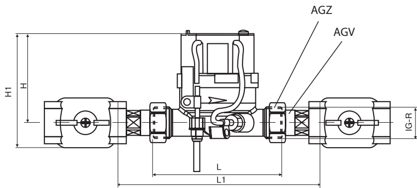
Рис. 4. Габаритные размеры теплосчетчика
