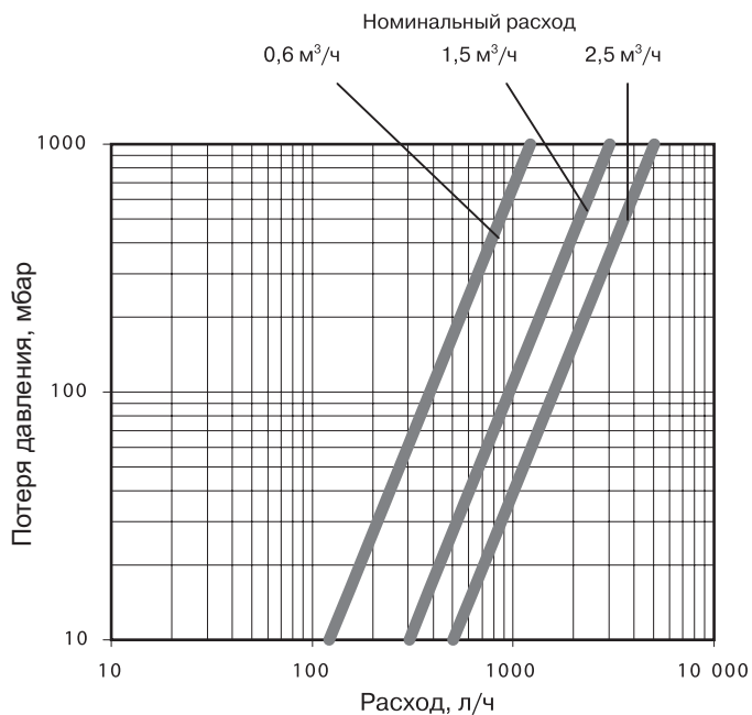
Рис. 3. Диаграмма потерь на теплосчетчике
