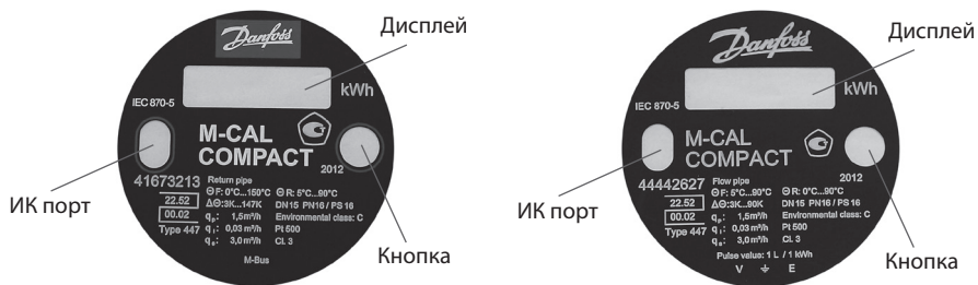
Рис. 5. Лицевая панель теплосчетчика
