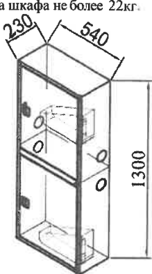
Рис. 1 Шкаф навесной закрытый правый с евро-замком
