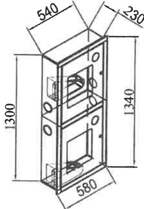
Рис. 2 Шкаф встроенный открытый левый
