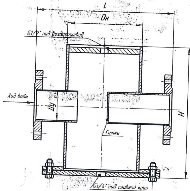
2 Исполнение фланцевое
