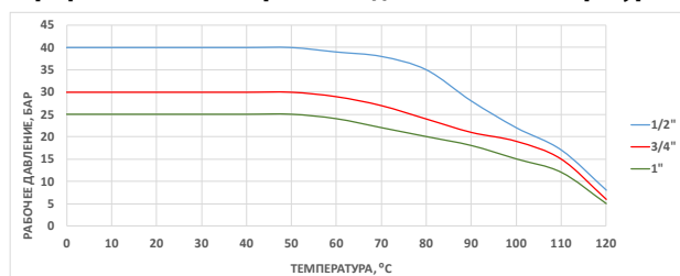
График зависимости рабочего давления от температуры
