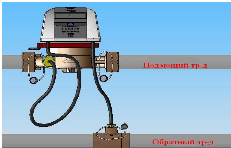
Рис.3 Монтаж теплосчетчика (монтаж термопреобразователя сопротивления в тройнике)
