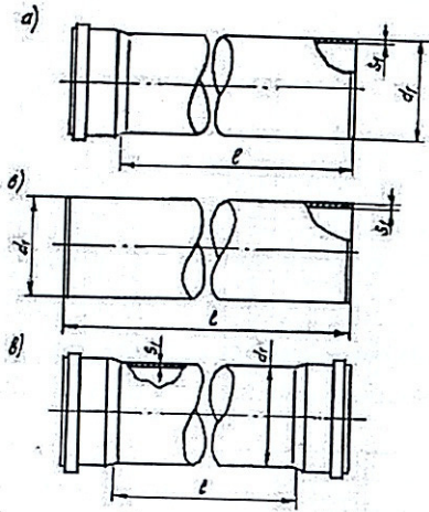
Рисунок 1. Трубы.
