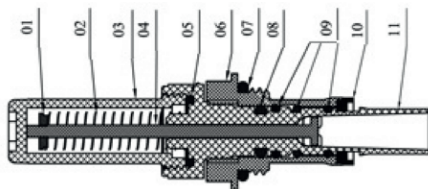
Конструкция и спецификация материалов расходомера коллектора 9501
