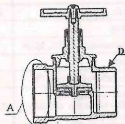
Клапан муфтово-цапковый
