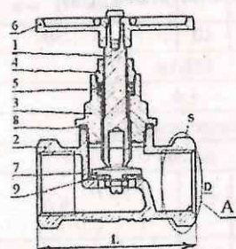
Клапан муфтовый
