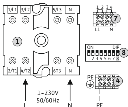
Fig. 4: Подключение к сети 1~230 В с главным выключателем
