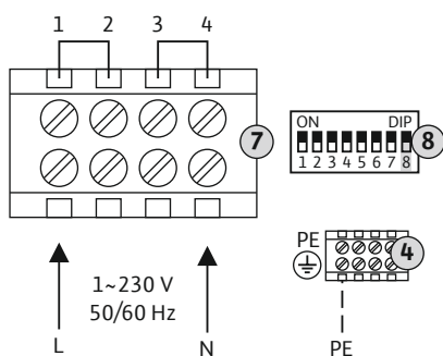
Fig. 6: Подключение к сети 1~230 В без главного выключателя
