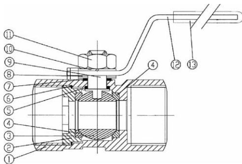
Рис. 4. Устройство крана шарового типа X1666
