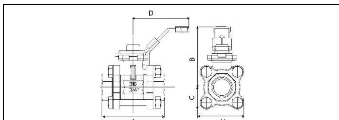
Рис. 36. Габаритные размеры кранов шаровых типов Х3900, Х3900В.
