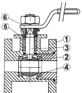
Рис. 16. Устройство крана шарового типа X2900F.
