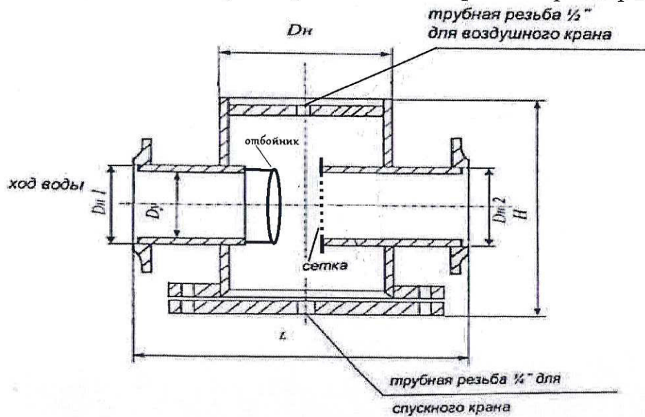
Фланцевое исполнение
