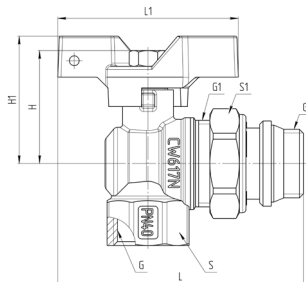
Рисунок 2 – Габаритные размеры крана.
