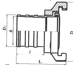
Рисунок 1. Головка напорная типа ГР.
