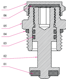
Конструкция и спецификация материалов балансировочного клапана коллектора 9504
