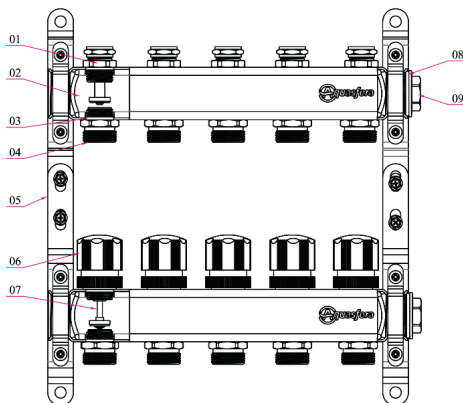
Конструкция и спецификация материалов коллекторной группы 9504
