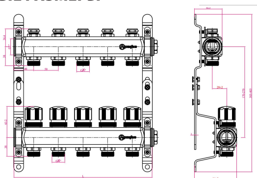
Габаритные и присоединительные размеры коллекторных групп 9504 Aquasfera
