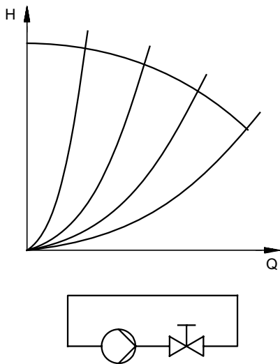
Рис. 8 Характеристика закрытой системы
