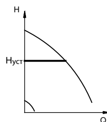
Рис. 16 Регулируемый режим – на примере регулирования по постоянному перепаду давления
