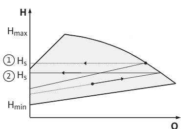
Fig. 39: Regulacja \Delta p -c/ \Delta p -v
