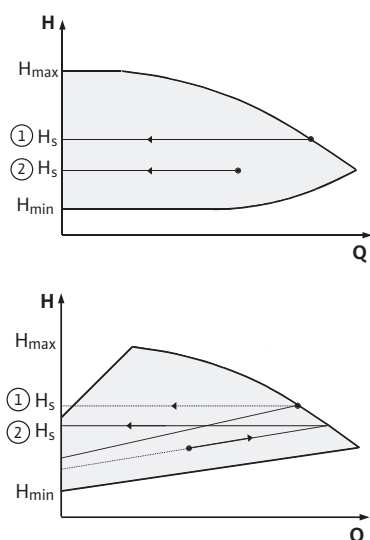
Fig. 39: Säättö \Delta p-c/\Delta p-v
