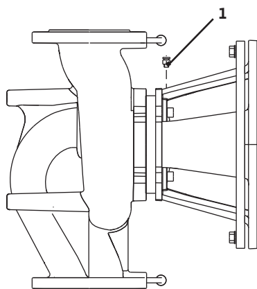
Fig. 37: Zawór odpowietrzający
