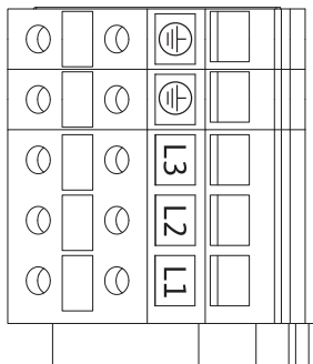
Fig. 22: Przyłączeniowe zaciski sieciowe
