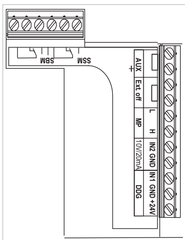
Fig. 21: Zaciski sterujące
