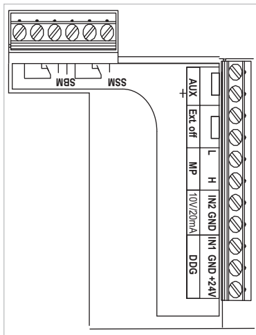
Fig. 21: Ohjausliittimet
