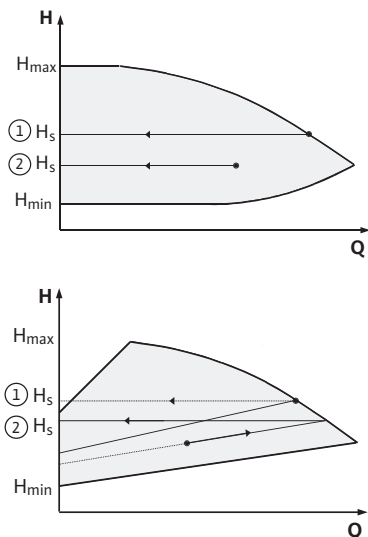
fig. 39: Reglering \Delta p-c/\Delta p-v
