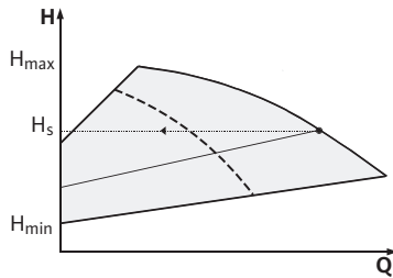
Рис. 15: Регулирование \Delta p -v (работа двух насосов)
